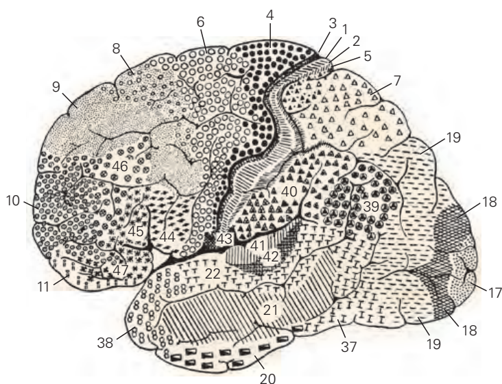
图 1.3.2: 20 世纪初，人类大脑皮层被分为 52 个独立的功能区。显示的区域是由解剖学家布罗德曼根据独特的神经细胞结构和细胞层的特征排列确定的。该方案至今仍在广泛使用，并不断更新。布罗德曼定义的几个区域被发现可以控制特定的大脑功能。例如，区域 4 是运动皮层，负责自主运动。区域 1、2 和 3 构成初级体感皮层，主要从皮肤和关节接收感觉信息。第 17 区是初级视觉皮层，它接收来自眼睛的感觉信号并将它们传递到其他区域以进行进一步处理。区域 41 和 42 构成初级听觉皮层。该图仅显示了皮层外表面的可见区域。
