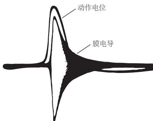
图 10.1.1: 动作电位由轴突膜离子电导的增加引起。肯尼思·科尔和霍华德·柯蒂斯于 1939 年进行的一项实验的历史记录显示了动作电位的示波器记录叠加在轴突膜电导的同步记录上。
