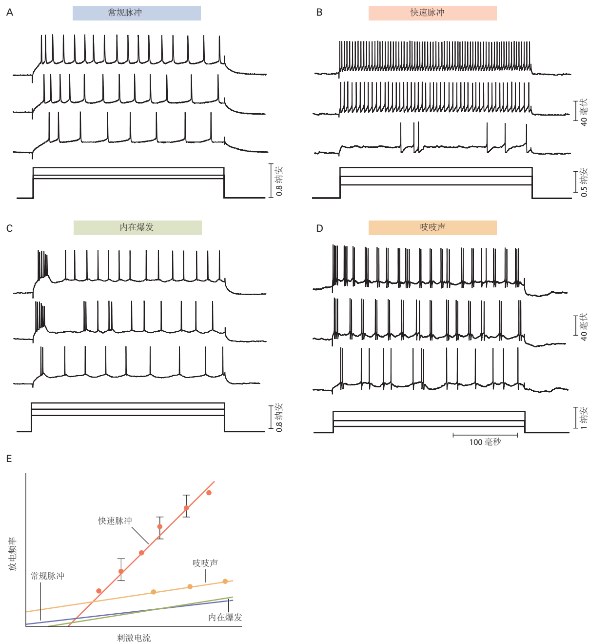
图 10.6.1: 4 种皮层神经元的不同放电模式。3 个步骤的去极化电流，每个具有不同的振幅，被注入每个细胞以引起放电 [60] 。A. 具有许多谷氨酸能皮层锥体神经元典型放电模式的皮层神经元，说明了适应性特征。B. 许多 \gamma -氨基丁酸能中间神经元的典型放电模式，说明维持高频重复放电。C. 在内在爆发的神经元中放电，这是皮层 II/III 中锥体神经元的一种亚型。D. 在震动细胞中放电，这是皮层 V 中锥体神经元的一种亚型。E. 这 4 种细胞类型的激发频率与刺激电流的关系，显示出它们对增加刺激强度的不同敏感性。
