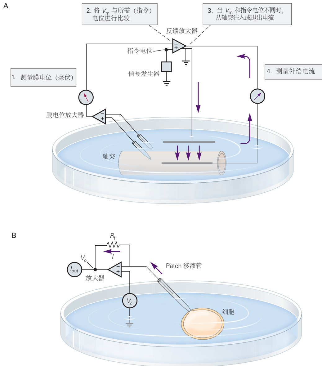
图 10.1.2: 电压钳的负反馈机制。A. 膜电位 ( V_m ) 由 2 个电极测量, 一个电极位于细胞内, 另一个电极位于槽内, 并与放大器相连。膜电位信号显示在示波器上, 并输入反馈放大器的负极端子。命令电位由实验者选择, 并且可以是任何期望的幅度和波形, 被馈送到反馈放大器的正端子。反馈放大器从指令电位中减去膜电位, 并放大这 2 个信号之间的任何差。放大器的电压输出连接到内部电流电极, 这是一根延伸轴突核心长度的细线。B. 使用膜片钳放大器的全细胞模式对神经元细胞体进行电压钳。贴片移液管密封在细胞上, 移液管下的膜破裂, 从而在细胞内部和移液管之间提供电连续性。移液管中的电极控制 V_m , 放大器通过反馈电阻器 ( R_f ) 提供电流 ( I ), 以将电极 (并因此将移液管溶液和细胞内部) 箝位到施加到另一放大器输入的命令电压 ( V_c )。放大器输出上的电压 ( V_o ) 与流过电极和膜的电流成比例。
