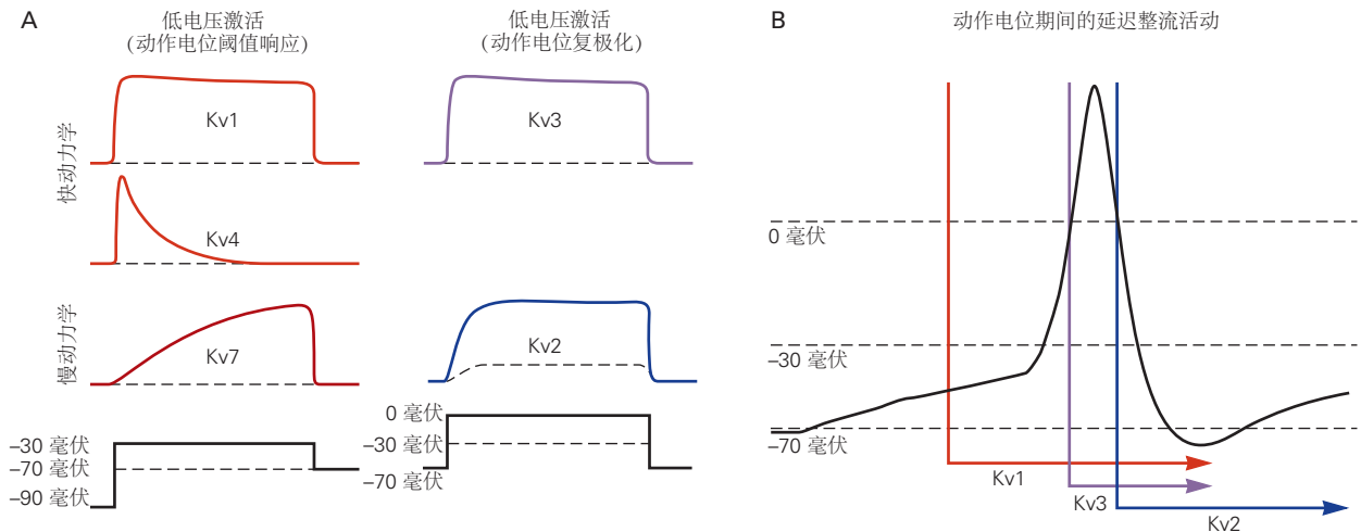
图 10.4.3: 哺乳动物电压激活 \text{K}^+ 通道主要类别的不同电压门控和动力学。A. 主要电压门控 \text{K}^+ 家族的电压门控和动力学的简化概括。由于 Kv1、Kv4 和 Kv7 通道可以被相对较小的去极化激活，因此它们通常有助于控制动作电位阈值。Kv2 和 Kv3 通道需要更大的去极化才能被激活。Kv1、Kv3 和 Kv4 通道的激活速度相对较快，而 Kv7 和 Kv2 通道的激活速度较慢。B. 动作电位期间延迟整流 \text{K}^+ 通道主要成分的不同激活时间的简化概括。Kv1 通道需要小的去极化并且被迅速激活，有时甚至比动作电位显著提前。Kv3 通道需要大的去极化，并且在动作电位的上升阶段后期被激活，此后非常迅速失活。Kv2 通道在动作电位下降阶段相对缓慢地被激活，并在后超极化期间保持开放 [59] 。
