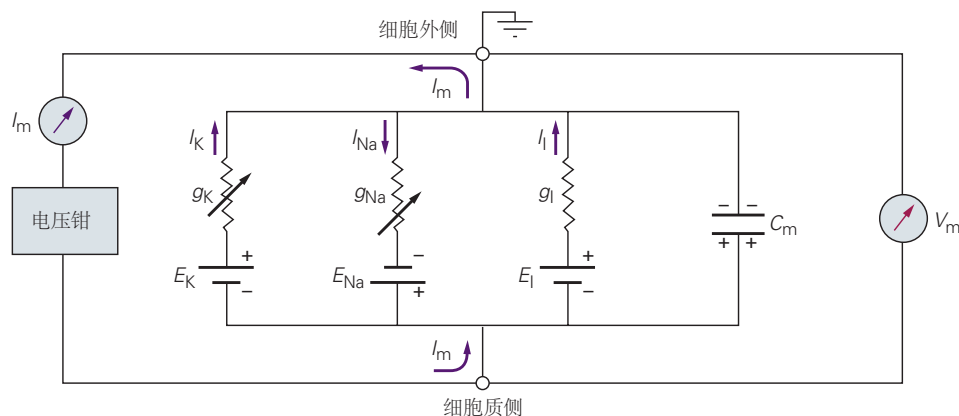
图 10.1.5: 电压钳神经元的等效回路。电压门控电导通路 ( g_{\text{K}} 和 g_{\text{Na}} ) 用可变电导的符号表示，即带有箭头的导体（电阻器）。电导是可变的，因为它依赖于时间和电压。这些电导与代表 \text{Na}^+ 和 \text{K}^+ 化学梯度的细胞串联。此外，泄漏电流 ( g_l 和 E_l ) 和电容电流 ( C_m ) 也有并行的通路。箭头表示激活 g_{\text{K}} 和 g_{\text{Na}} 的去极化步骤中的电流。
