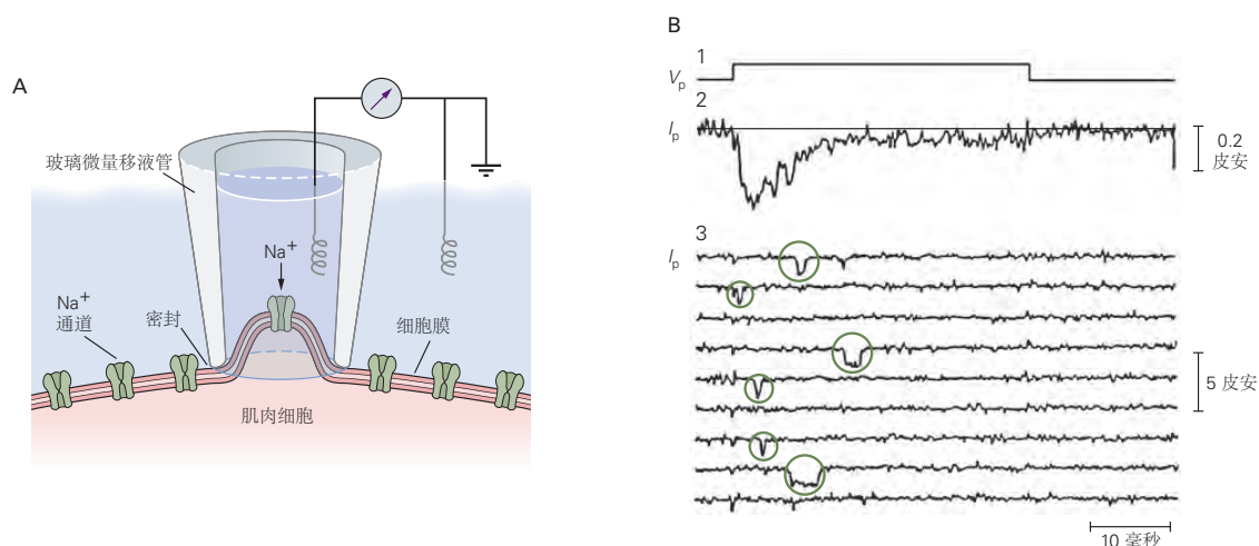
图 10.2.1: 各个电压门控离子通道以全有或全无的方式打开。A. 一小块包含单个电压门控 \text{Na}^+ 通道的膜通过贴片电极与细胞的其余部分电隔离。通过通道进入细胞的 \text{Na}^+ 电流由连接到贴片电极的监视器记录（见文本框 8.1）。B. 培养的大鼠肌肉细胞中单个 \text{Na}^+ 通道的记录。（1）在隔离的膜片上施加 10 毫伏去极化电压阶跃的时间过程（ V_p = 膜片上的电位差）。（2）在 300 次试验期间通过贴片中 \text{Na}^+ 通道的内向电流总和（ I_p 是通过贴片的电流）。通过用四乙铵封闭 \text{K}^+ 通道并以电子方式减去泄漏电流和电容电流来获得迹线。（3）300 组中的 9 个单独试验，显示通道的 6 个开口（圆圈）。如图 10.1.3B 所示，这些数据表明，传统电压钳记录中记录的总 \text{Na}^+ 电流可以通过大量 \text{Na}^+ 通道的全开或关闭的统计性质来解释 [52] 。
