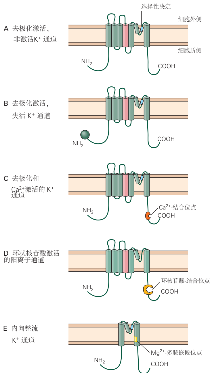
图 10.4.1: 电压门控通道的扩展基因家族产生了常见分子设计的变体。A. 电压门控 K^+ 通道的 \alpha 亚基的基本跨膜拓扑结构。S4 跨膜 \alpha -螺旋标记为红色。B. 许多首先被激活然后因长时间去极化而失活的 K^+ 通道在其 N 末端有一个球链片段, 通过堵塞通道的内口使通道失活。C. 一些需要去极化和细胞内 Ca^{2+} 增加才能激活的 K^+ 通道具有连接到通道 C 末端的 Ca^{2+} 结合序列。D. 由环核苷酸门控的阳离子通道具有连接到 C 末端的环核苷酸结合域。此类通道的一个子类包括在嗅觉和视觉感觉信号的转导中很重要的电压门控、环核苷酸门控通道。如图 10.4.2D 所示, 另一个子类包括对起搏器活动很重要的超极化激活环核苷酸门控阳离子通道。这些通道中的 P 环缺乏 K^+ 选择性所需的关键氨基酸残基。因此, 这些通道对 Na^+ 和 K^+ 没有显示出高度的区分度。E. 内向整流 K^+ 通道由细胞质中可用的阻断颗粒门控, 由基本构建块的截短版本形成, 只有 2 个跨膜区域和 1 个 P 区域。
