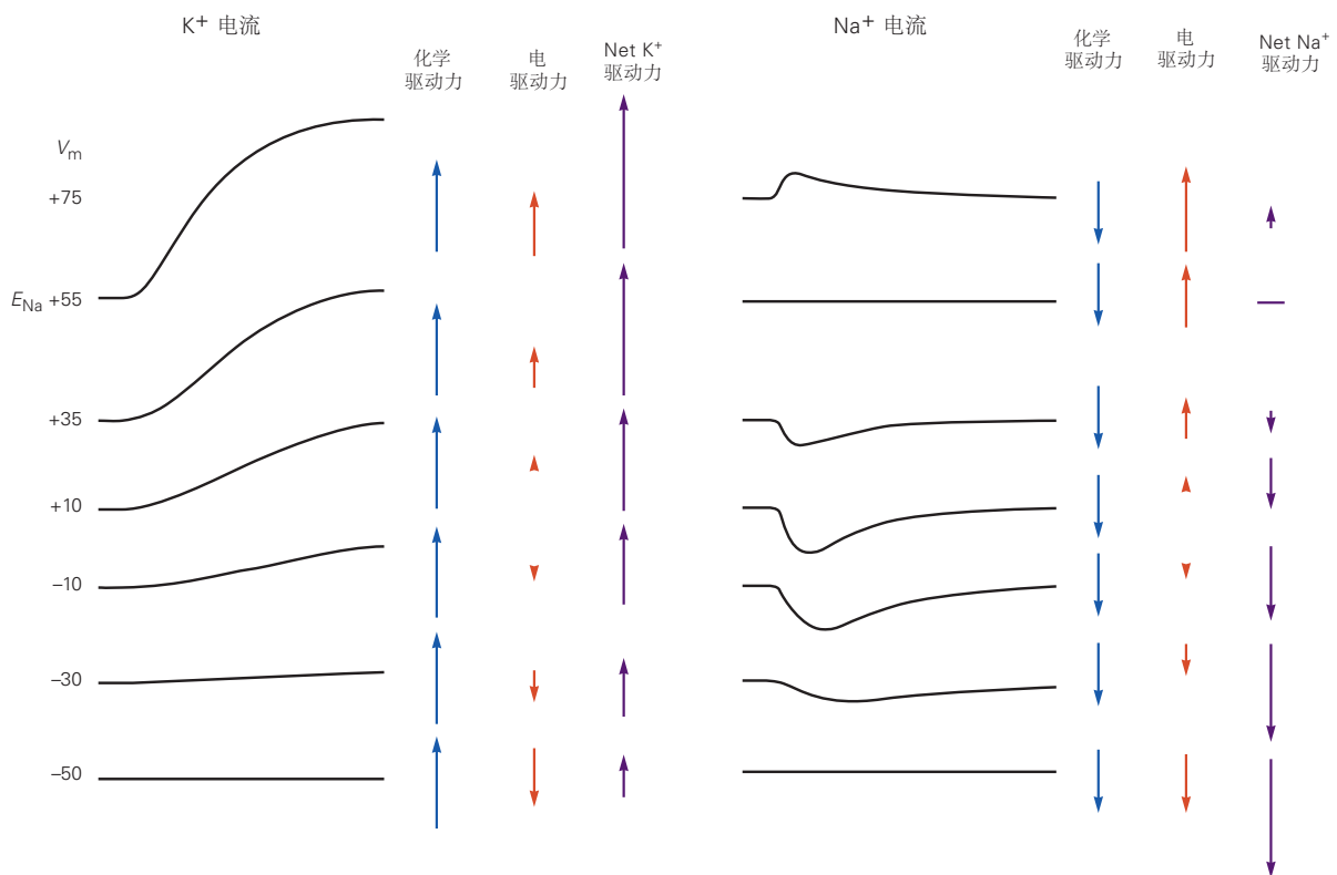
图 10.1.4: 钠和钾膜电流的大小和极性随膜去极化的幅度而变化。左：随着渐进去极化，电压钳位膜 K^+ 电流单调增加，因为 g_K 和 (V_m E_K) ， K^+ 的驱动力，随着去极化的增加而增加。去极化期间的电压显示在左侧。 K^+ 上的化学 ( E_K ) 和电驱动力的方向和大小（以及净驱动力）由每条迹线右侧的箭头给出（向上箭头表示向外力；向下箭头表示向内力）。右图：起初，由于 g_{Na} 的增加， Na^+ 电流变得越来越向内，去极化也越来越大。然而，当膜电位接近 E_{Na} (+55 毫伏) 时，由于内向驱动力 ( V_m E_{Na} ) 的减少，内向 Na^+ 电流的幅度开始减小。最终，当膜电位达到 E_{Na} 时， I_{Na} 变为 0。在对 E_{Na} 正去极化时，( V_m E_{Na} ) 的符号反转并且 I_{Na} 向外。
