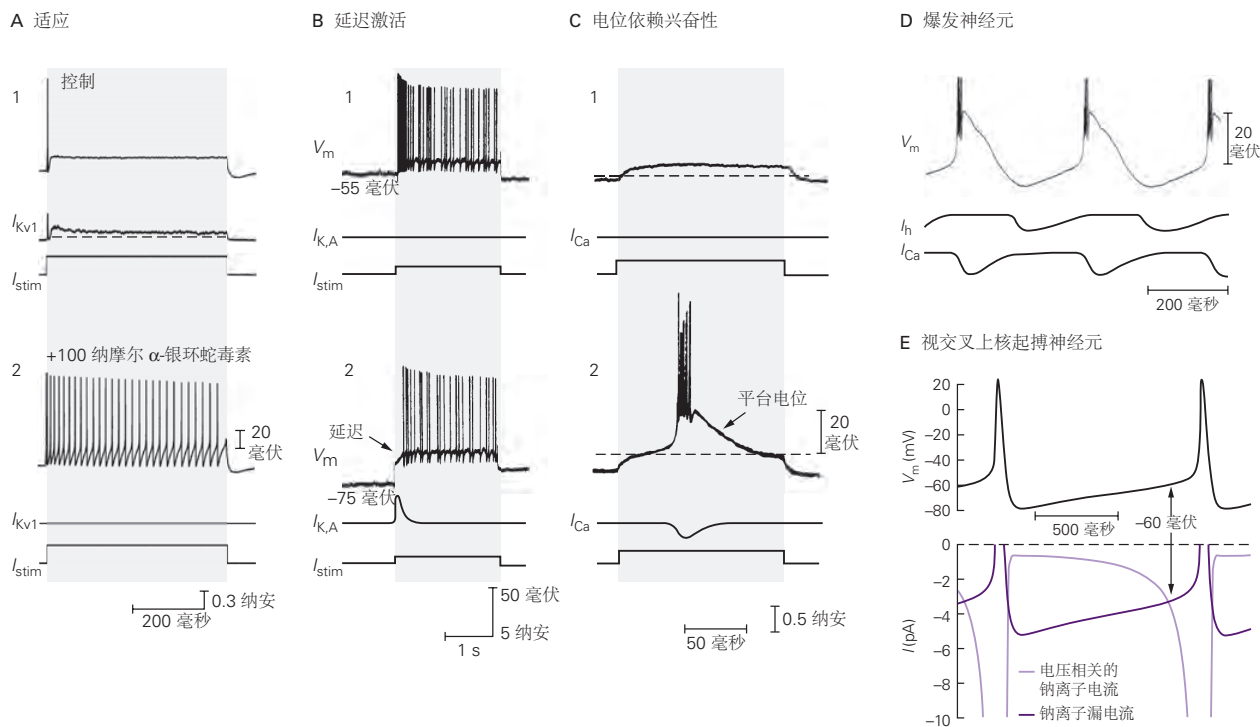
图 10.4.2: 通过各种电压门控通道调节激活模式。A. Kv1 通道的激活通常通过增加小鼠背根神经节神经元中的脉冲阈值来阻止第二动作电位的激活 (1)。用蛇毒素 \alpha -树毒素阻断 Kv1 通道可将激发模式从强烈适应改变为响应稳定刺激电流 ( I_{stim} ) 的持续重复激发 (2)。B. 将去极化电流脉冲 ( I_{stim} ) 注入孤束核中的神经元通常会立即触发一系列动作电位 (1)。如果细胞首先保持在超极化膜电位，则脉冲序列会延迟 (1)。延迟是在 A 型 K^+ 通道被去极化电流脉冲激活时引起的。这些通道产生一个瞬态外向 K^+ 电流 I_{K,A} ，它会短暂地减慢 V_m 接近阈值的速率。这些通道通常在静息电位 (-55 毫伏) 下失活，但稳定的超极化消除了失活 [55] 。C. 注入静止的丘脑神经元的小去极化电流脉冲会产生亚阈值去极化 (1)。如果膜电位保持在超极化水平，则相同的电流脉冲会触发动作电位的爆发 (2)。电流脉冲的有效性得到增强，因为超极化导致一种电压门控 Ca^{2+} 通道从失活中恢复。通过这些 Ca^{2+} 通道 ( I_{Ca} ) 去极化内向电流会产生约 20 毫伏的平台电位，触发动作电位爆发。虚线表示正常静息电位的水平 [56] 。B 部分和 C 部分的数据表明：稳定的超极化（例如可能由神经元的抑制性突触输入产生）可以深刻影响神经元的脉冲序列模式。这种效应在细胞类型之间差异很大，取决于特定类型的电压门控 Ca^{2+} 和 K^+ 通道的存在与否。D. 在没有突触输入的情况下，丘脑皮层中继神经元可以在动作电位的短暂爆发中自发放电。这些爆发由电流通过 2 种类型的电压门控离子通道产生。导致爆发的逐渐去极化由通过超极化激活环核苷酸门控阳离子通道的内向电流 ( I_h ) 驱动，该通道响应超极化而打开。爆发由通过电压门控 Ca^{2+} 通道 3 的内向 Ca^{2+} 电流触发，这些通道在相对较低的去极化水平下被激活。这种 Ca^{2+} 流入产生足够的去极化以达到阈值并驱动 Na^+ -依赖性动作电位的短暂爆发。爆发期间的强烈去极化导致超极化激活环核苷酸门控阳离子通道关闭并使 Ca^{2+} 通道失活，从而允许超极化在发射爆发之间发展。这种超极化然后打开超极化激活环核苷酸门控阳离子通道，启动下一个节律循环 [57] 。E. 来自下丘脑视交叉上核的神经元产生自发的起搏电位。在动作电位之后，神经元自发地去极化，首先缓慢然后更快，从而产生另一个动作电位。在脉冲间期，去极化由 2 个内向的 Na^+ 电流驱动。一种是“持续的 Na^+ 电流”，它流经对河豚毒素阻断敏感的电压门控 Na^+ 通道，可能与动作电位上升过程中更大的 Na^+ 电流背后的通道群相同。第二个电流流经非电压激活钠泄漏非选择性通道，该通道为 Na^+ 和 K^+ 提供稳定的电导通路。在负电压下， Na^+ 驱动力大而 K^+ 驱动力小，因此漏电流主要由 Na^+ 携带。这种内向电流使神经元去极化，使电压门控持久 Na^+ 电流成为主导（约 -60 毫伏） [58] 。
