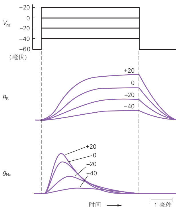
图 10.1.6: K^+ 通道和 Na^+ 通道对长时间去极化的响应。增加去极化引起 K^+ 电导 g_K 和 Na^+ 电导 g_{Na} 的分级增加, 这反映了数千个电压门控 K^+ 和 Na^+ 通道的比例开放。 Na^+ 通道比 K^+ 通道打开得更快。在维持去极化过程中, 由于失活门的关闭, Na^+ 通道在打开后关闭。 K^+ 通道保持开放状态是因为它们缺乏快速灭活过程。在非常正的 V_m 下, K^+ 和 Na^+ 电导接近最大值, 因为去极化足以打开几乎所有可用通道。
