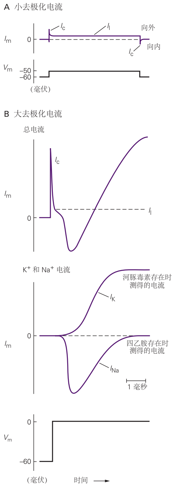
图 10.1.3: 电压钳实验演示了电压门控 Na^+ 通道和 K^+ 通道的顺序激活。A. 小的去极化（10 毫伏）会引发电容电流 I_c 和漏电流 I_l ，它们是总膜电流 ( I_m ) 的组成部分。B. 较大的去极化（60 毫伏）会导致较大的电容电流和漏电流，以及随时间变化的内向离子电流和随时间变化的外向离子电流。顶部：响应去极化的总（净）电流。中间：单独的 Na^+ 电流和 K^+ 电流。在存在阻断 Na^+ 电流的河豚毒素或存在阻断 K^+ 电流的四乙胺的情况下使细胞去极化，显示减去后的纯 K^+ 和 Na^+ 电流（分别为 I_K 和 I_{Na} ） I_c 和 I_l 。底部：电压阶跃。
