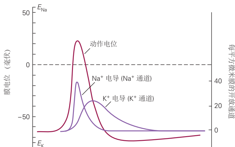
图 10.1.7: 电压门控 \text{Na}^+ 和 \text{K}^+ 通道的顺序打开会产生动作电位。霍奇金和赫胥黎的一项伟大成就是将动作电位期间电导的变化分解为可归因于 \text{Na}^+ 和 \text{K}^+ 通道开放的独立成分。动作电位的形状和潜在的电导变化可以根据电压门控 \text{Na}^+ 和 \text{K}^+ 通道的特性来计算 [51] 。
