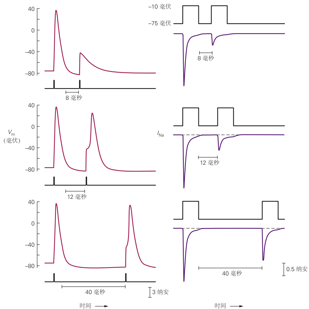
图 10.1.8: 不应期与 \text{Na}^+ 通道从失活中恢复有关。左图：小鼠背根神经节神经元对 2 个电流脉冲的电压响应（底部迹线）。第一个触发动作电位；第二个触发可变电电压响应，具体取决于电流脉冲之间的延迟。右图：由 2 个去极化电压脉冲引起的同一个细胞在电压钳下记录的钠电流，2 个去极化电压脉冲由左侧记录中指示的间隔分开。在这个神经元中，不应期对应于恢复大约 20% 的 \text{Na}^+ 通道所需的时间。
