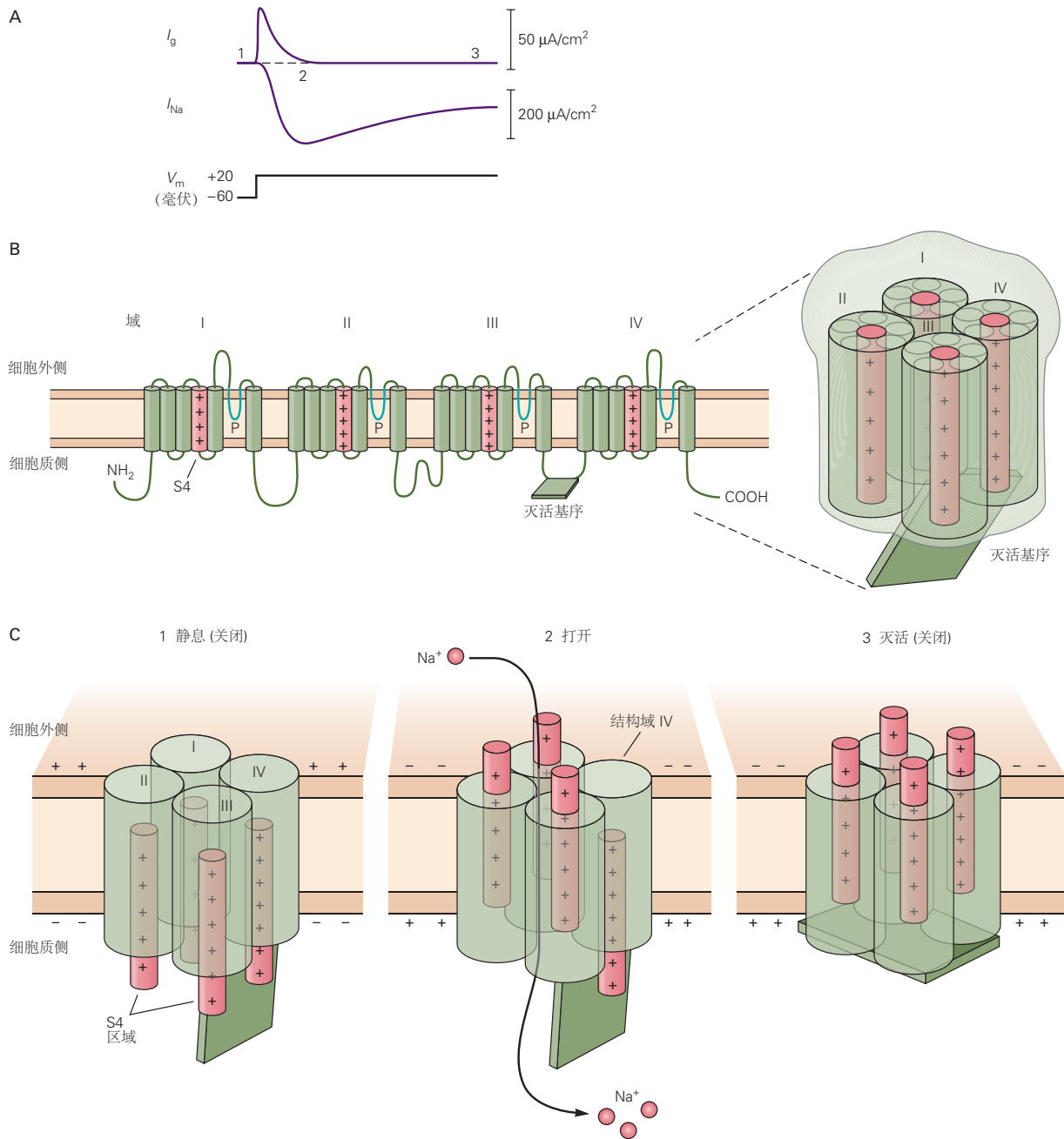
图 10.2.2: Na + 通道的打开和关闭与电荷的重新分配有关。A. 当膜去极化时, Na + 电流 ( I_{Na} ) 被激活然后失活。Na + 电流的激活之前是一个短暂的电容性门控电流 ( I_g ), 反映了正电荷在 Na + 通道壁内向外移动。为了检测这个小的门控电流, 有必要阻止离子电流流过 Na + 和 K + 通道, 并减去使脂质双层去极化的电容电流 [53] 。B. 哺乳动物 Na + 通道 \alpha -亚基的二级结构显示门控电荷的位置。Na + 通道 \alpha 亚基是由 4 个重复结构域组成的单一多肽, 每个结构域包含 6 个跨膜区域。每个结构域的第四个跨膜区 (S4 区) 包含带正电的精氨酸和赖氨酸残基, 它们形成通道的门控电荷 [54] 。C. 图表描绘了当通道处于静止、打开和失活状态时, 门控电荷的重新分布以及激活和失活门的位置。红色圆柱体代表包含正门控电荷的 S4 区域。细胞膜从静止状态去极化导致门控电荷向外移动。结构域 I、II 和 III 的 S4 区域向外运动与激活相关 (1-2), 而结构域 IV 的 S4 区域较慢的运动与失活相关 (2-3)。结构域 IV 的 S4 区域的移动允许结构域 III 和 IV 之间的细胞内环 (描绘为绿色矩形) 结合到孔内部 S6 螺旋附近的停靠位点, 变构地稳定失活的闭合状态 [54] 。
