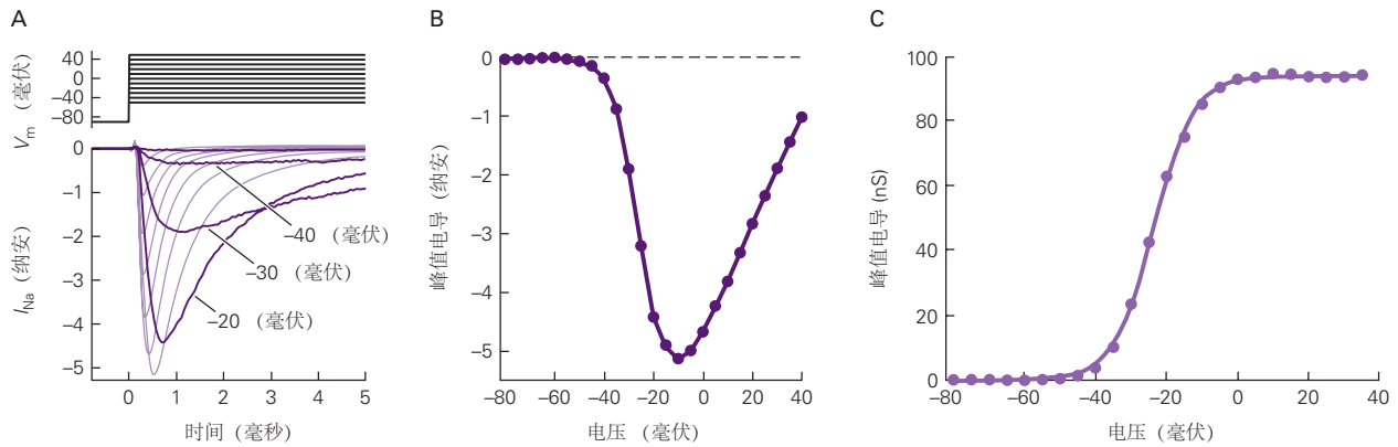
图 10.2.3: Na + 通道激活的电压门控由门控电荷的数量决定。A. 在分离的海马锥体神经元中进行电压门控 Na + 电流的全细胞膜片钳记录。通过阻断通过 K + 和 Ca 2+ 通道的电流，然后减去阻断 Na + 电流后剩余的电容电流和漏电流，从而隔离 Na + 通道电流。B. 峰值 Na + 电流的电流-电压曲线。C. 峰值 Na + 电导与膜电位。如文本框 10.2 所示，根据峰值电流计算出响应一系列去极化电压阶跃的峰值 g_{Na} 增加。实验数据点符合玻尔兹曼关系，形式为 g_{Na}/g_{Na(max)} = 1/[1 + \exp(-(V_m - V_h)/k)] ，其中 V_h = 24 毫伏是激活曲线的中点， k = 5.5 是“斜率因子”，单位为毫伏， g_{Na(max)} 是正电压下的最大钠电导。打开通道必须移动的门控电荷数量越多，斜率因子就越小。大多数电压门控通道的电压门控可以通过类似的玻尔兹曼曲线来拟合。
