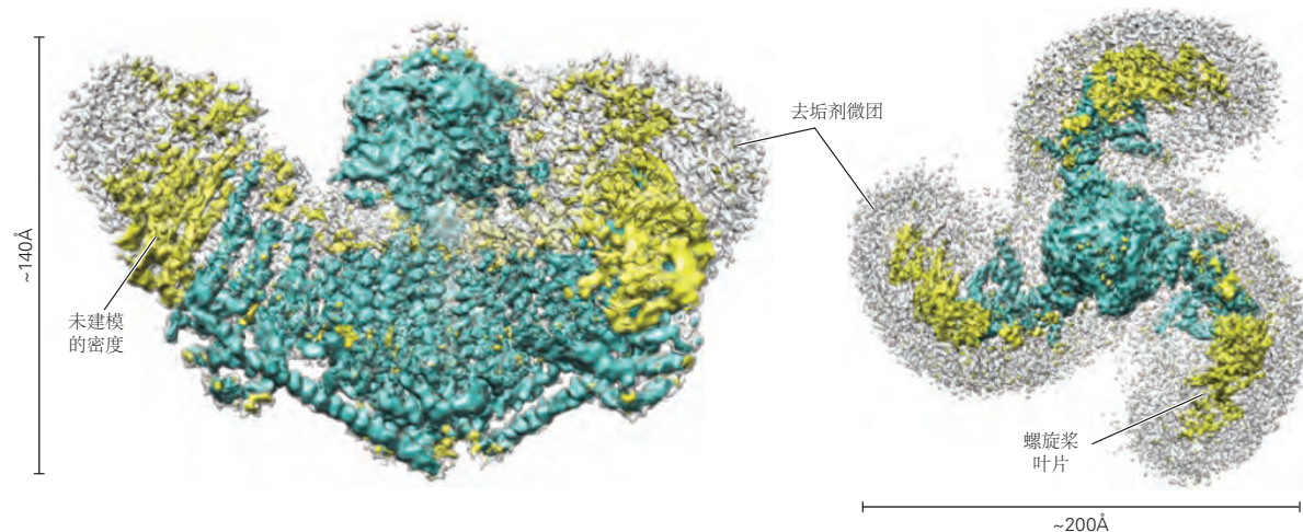
图 18.3.2: 压电型机械敏感离子通道组件 1 离子通道的结构和分子组织。A. 压电型机械敏感离子通道组件 1 和压电型机械敏感离子通道组件 2 具有同源蛋白质结构，包含大约 2,500 个氨基酸，至少有 26 个假定的跨膜片段。它们组合成三聚体，形成哺乳动物体内最大的膜离子通道 [143] 。B. 从低温电子显微镜推断出的压电型机械敏感离子通道组件 1 离子通道的推定结构。1. 侧面观，胞浆面朝下。2. 从细胞外侧俯视图。受体是由 3 个相同的压电型机械敏感离子通道组件 1 亚基组成的三脚架。3 种压电蛋白的 C 端形成一个中央细胞外帽，连接到跨膜孔的细胞外表面，跨膜孔延伸到膜外进入细胞质尾区。穿过通道的水孔延伸穿过帽的中心轴、跨膜孔和细胞质尾区。3 个蛋白质亚基的 N-末端排列在外围，形成螺旋桨状的螺旋结构。蓝色表示高分辨率建模区域 [144] 。
