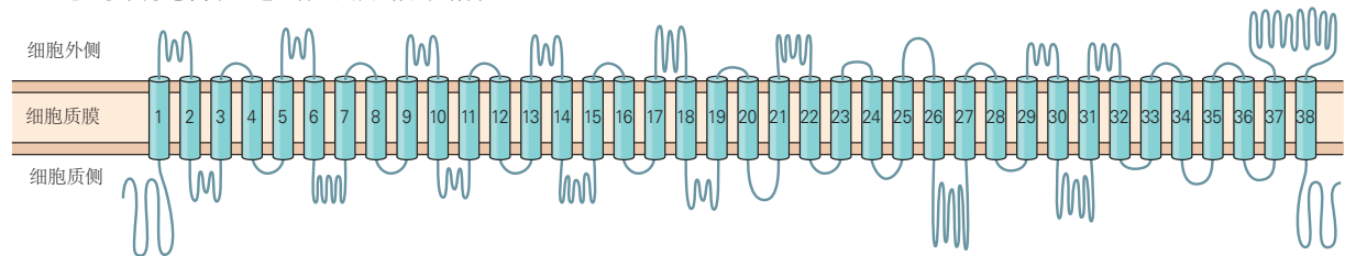
A 压电型机械敏感离子通道组件1 蛋白的分子结构
