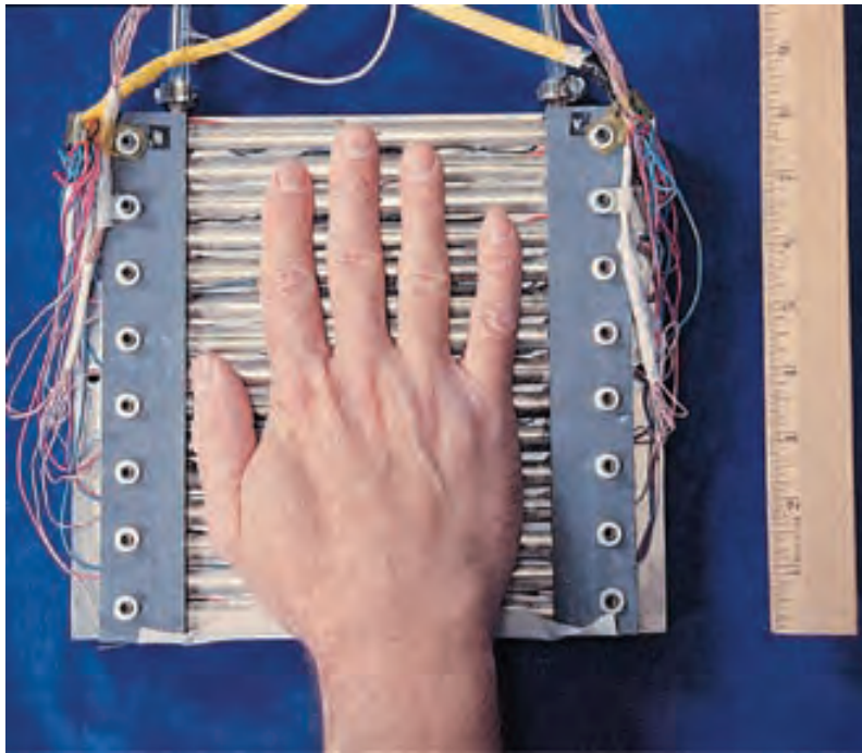
图 20.6.1: 桑伯格的烤架。刺激表面 ( 20 \times 14 厘米) 由 15 根纯银条制成，每条宽 1 厘米，间隔约 3 毫米。在每个棒的下面是 3 个纵向间隔的热电 (帕尔贴) 元件 ( 1\text{cm}^2 )，在每个棒上是一个热电偶。交替 (偶数和奇数) 条可以独立控制 [183] 。
