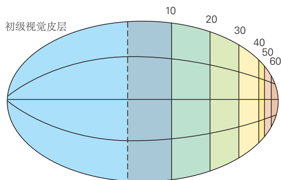
图 21.4.3: 感受野大小、偏心率、视网膜组织和放大倍数。颜色编码指的是视觉空间或视网膜上的位置。A. 感受野与中央凹的距离称为感受野的偏心率。B. 感受野大小随与中央凹的距离而变化。最小的视场位于注视中心（即中央凹）视觉分辨率最高；视场随着距中央凹的距离逐渐变大。C. 专用于每个视觉空间度数内输入的皮层区域的数量，称为放大因子，也随偏心率而变化。视野的中央部分控制着最大的皮层区域。例如，在初级视觉皮层中，更多的区域专用于视觉空间的中心 10^\circ ，而不是其他所有区域。初级视觉皮层的映射显示皮层片展开。
