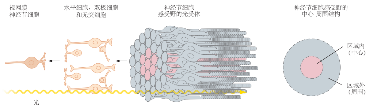
图 21.4.1: 与光受体相关的视网膜神经节细胞的感受野。A. 对视网膜神经节细胞感受野有贡献的光受体数量因感受野在视网膜上的位置而异。如图 21.4.3 所示，中央凹附近的细胞接收来自覆盖较小区域的较少受体的输入，而远离中央凹的细胞接收来自覆盖较大区域的更多受体的输入。B. 光线穿过神经细胞层到达视网膜后部的光受体。来自光受体的信号随后由外核层和内核层中的神经元传输到视网膜神经节细胞。
