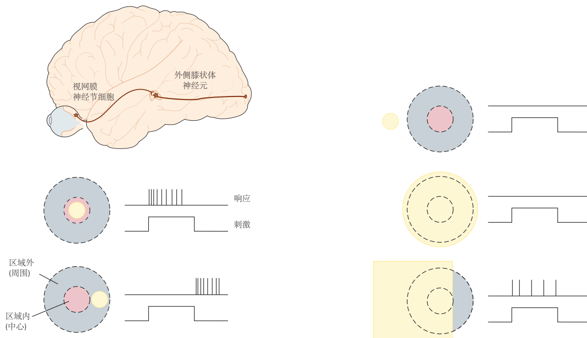
图 21.4.2: 视觉通路早期中继神经元的感受野。具有相互对立的中心和周围的圆形对称感受野是丘脑外侧膝状体核中视网膜神经节细胞和神经元的特征。中心可以响应光点（黄色）的打开或关闭，具体取决于感受野分别属于“在中心”还是“偏离中心”类。环绕有相反的反应。在环绕之外，对光没有响应，从而定义了感受野边界。当光线同时覆盖中心和周围时，响应较弱，因此这些神经元对视野中的对比度（明暗边界）做出最佳响应。
