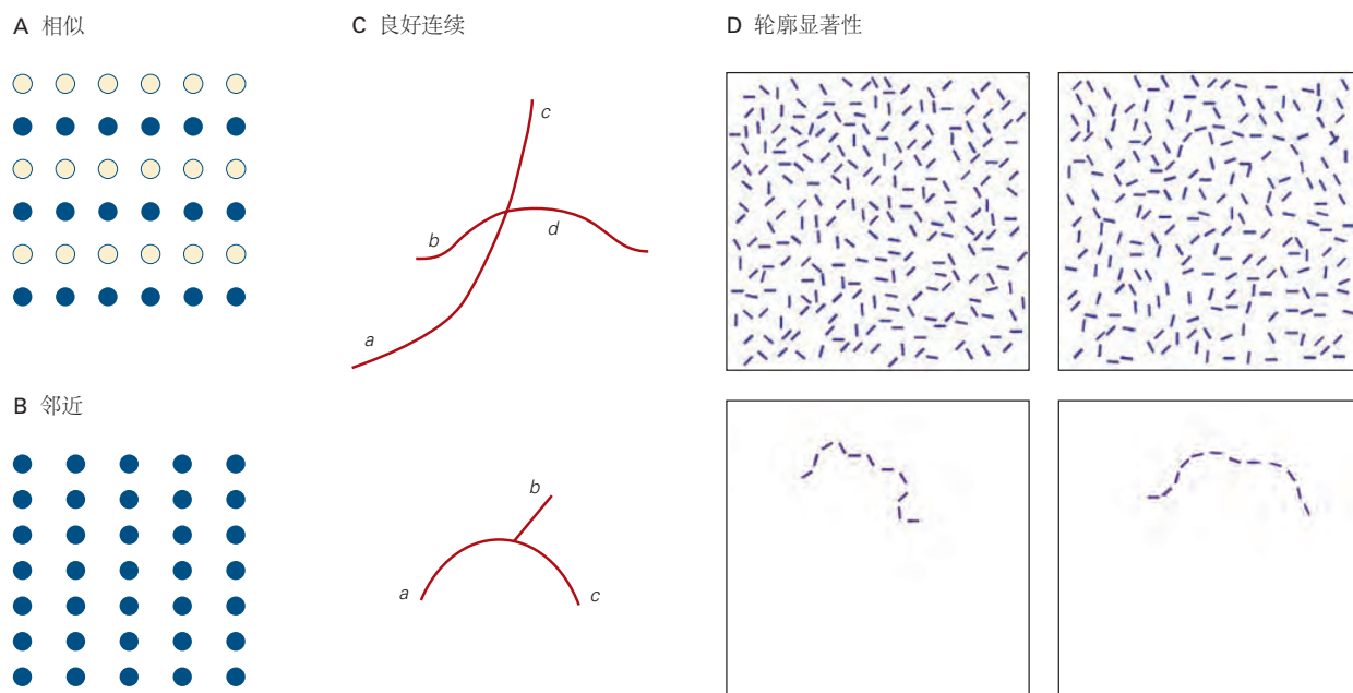
图 21.1.1: 视觉感知的组织规则。为了将视觉场景的元素连接成统一的感知，视觉系统依赖于组织规则，如相似性、邻近性和良好的连续性。A. 因为交替行中的点具有相同的颜色，所以整体图案是蓝色和白色行。B. 列中的点比行中的点靠得更近，导致列的感知。C. 当线段共线时，它们在感知上是相连的。在顶部的一组线中，人们更有可能将线段 a 视为属于 c 而不是 d。在底部集合中，a 和 c 在感知上是相关的，因为它们保持相同的曲率，而 a 和 b 似乎是不连续的。D. 良好连续性原则也见于轮廓显著性。在右侧，线条元素的平滑轮廓从背景中弹出，而左侧的锯齿状轮廓消失在背景中 [185] 。
