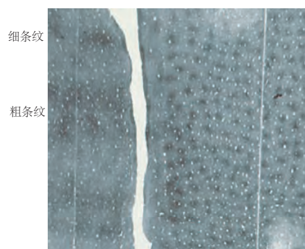
图 21.5.1: 初级视觉皮层的功能结构。A. 初级视觉皮层的表面在功能上被组织为视野映射。如图 21.4.3 所示，视觉空间的仰角和方位角被组织在一个规则的网格中，由于放大系数的变化而扭曲。此处的网格在深色条纹中可见（通过固有信号光学成像可视化），它反映了神经元对一系列垂直肯特直条纹做出响应的模式。在此表面图中，人们发现了功能特定的细胞柱的重复叠加循环，如 B、C 和 D. B 中所示。B. 深色和浅色条纹代表左右眼优势柱的表面视图。这些条纹以直角与区域初级视觉皮层和二级视觉皮层之间的边界成直角相交。C. 一些列包含对刺激方向具有相似选择性的细胞。不同的颜色表示柱的方向偏好。表面视图中的方向列最好描述为围绕方向突然变化奇点（风车中心）的风车。比例尺代表 1 毫米。D. 初级视觉皮层中的斑点图案和二级视觉皮层中的条纹代表功能组织的其他模块。这些模式用细胞色素氧化酶可视化。
