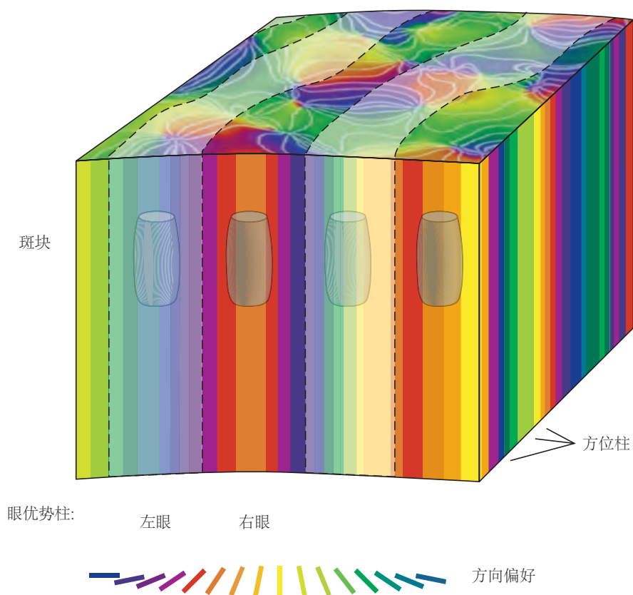
图 21.5.2: 皮层计算模块。一块大约 1 平方毫米的皮层组织包含一个定向超柱（一个完整的定向柱循环）、一个左眼和右眼优势柱循环，以及斑点和间斑。该模块可能包含初级视觉皮层的所有功能和解剖细胞类型，这些细胞将重复数百次以覆盖视野 [187] 。
