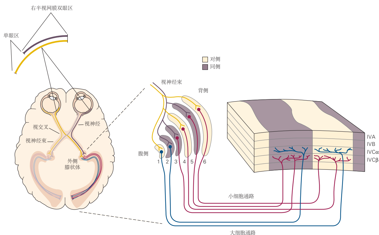
图 21.2.3: 从外侧膝状体到视觉皮层的投射。每个半球的外侧膝状体核接收来自同侧眼的颞侧视网膜和对侧眼的鼻侧视网膜的输入。细胞核是一种分层结构，包括 4 个小细胞层（第 3 至 6 层）和 2 个大细胞层（第 1 层和第 2 层）。每个都与插入的粒状层配对（如图 21.5.3 所示，这些层在这里由分隔主要层的间隙表示。它们没有标记以避免混乱）。来自两只眼睛的输入终止于不同的膝状体层：对侧眼投射到层 1、4、和 6，而同侧眼睛将输入发送到第 2、3 和 5 层。来自这些膝状体层的神经元然后投射到皮层的不同层。如图 21.5.3 和图 21.6.1 所示，小细胞膝状体神经元投射到 IVC \beta 层，大细胞神经元投射到 IVC \alpha 层，而粒状神经元投射到上皮层的“斑块”。此外，来自外侧膝状体同侧和对侧层的传入神经被分离到交替的眼优势柱中。
