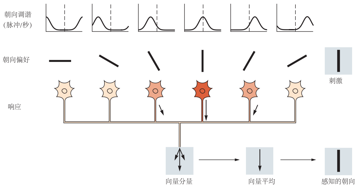
图 21.7.1: 向量平均是神经回路中群体编码的一种模型。向量平均值描述了神经元集合中的响应、集合中单个神经元的调谐特性以及由此产生的感知之间的可能关系。单个神经元对视野中刺激的特定方向做出最佳响应，但也会以不同的速率对一系列方向做出响应。神经元最能激发的刺激方向可以被认为是一个线标签，当细胞快速激发时，它的活动表示存在具有该方向的刺激。许多具有不同方向偏好的神经元会对相同的刺激做出响应。每个神经元的响应都可以表示为一个向量，其长度表示其响应的强度，其方向表示其偏好方向或线标签 [189] 。
