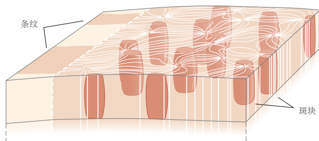
图 21.5.1: 初级视觉皮层的功能结构。A. 初级视觉皮层的表面在功能上被组织为视野映射。如图 21.4.3 所示，视觉空间的仰角和方位角被组织在一个规则的网格中，由于放大系数的变化而扭曲。此处的网格在深色条纹中可见（通过固有信号光学成像可视化），它反映了神经元对一系列垂直肯特直条纹做出响应的模式。在此表面图中，人们发现了功能特定的细胞柱的重复叠加循环，如 B、C 和 D. B 中所示。B. 深色和浅色条纹代表左右眼优势柱的表面视图。这些条纹以直角与区域初级视觉皮层和二级视觉皮层之间的边界成直角相交。C. 一些列包含对刺激方向具有相似选择性的细胞。不同的颜色表示柱的方向偏好。表面视图中的方向列最好描述为围绕方向突然变化奇点（风车中心）的风车。比例尺代表 1 毫米。D. 初级视觉皮层中的斑点图案和二级视觉皮层中的条纹代表功能组织的其他模块。这些模式用细胞色素氧化酶可视化。
