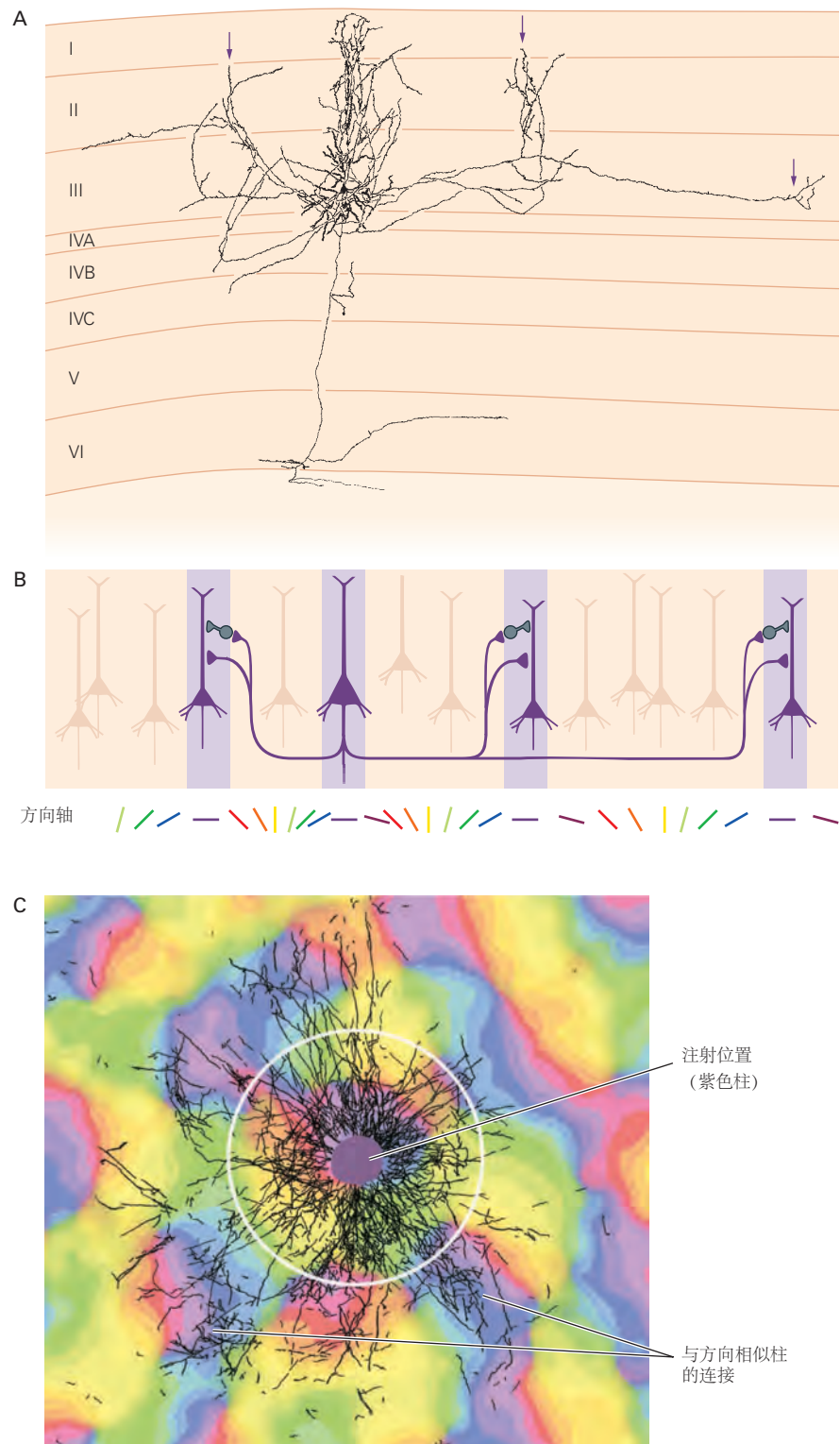
图 21.6.2: 视觉皮层每一层的远程水平连接整合了来自视野不同部分的信息。A. 锥体细胞的轴突平行于皮层表面延伸数毫米。轴突侧枝与其他锥体细胞以及抑制性中间神经元形成连接。这种安排使神经元能够整合大部分视野的信息。这些连接的一个重要特征是它们与功能柱的关系。在距离细胞体大于 0.5 毫米的距离处，轴突侧支呈簇状（箭头）。B. 水平连接将具有相似方向特异性的细胞列连接起来。C. 通过将包含绿色荧光蛋白编码基因的腺病毒载体注入一个定向柱并将标记图像（黑色）叠加在注射附近定向柱的光学成像图上，可以看到水平连接的模式（白色圆圈的直径为 1 毫米）。
