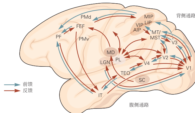
图 21.3.1: 大脑皮层中的视觉通路。A. 功能性核磁共振成像显示了人类大脑皮层参与视觉处理的区域。顶行显示大脑正常视图的脑回和脑沟区域；中间一行显示了大脑的“膨胀”视图，该计算过程模拟大脑像气球一样膨胀，以便将脑回和脑沟的“皱纹”拉伸成光滑的表面，同时最大限度地减少局部变形。浅灰色和深灰色区域分别代表脑回和脑沟；底行显示了枕叶的二维表示（左）和通过沿距状裂进行切割而失真较小的表示。划分不同的功能区域需要不同的方法。根据定义，视网膜区域包含视觉空间的连续图，并使用诸如旋转螺旋或扫过视觉空间的扩大圆圈等刺激来识别。相邻皮层区域的映射在皮层表面以相反的方向运行，并沿着局部镜像反转的边界相交。这些镜像反转可用于识别区域边界，从而划分每个区域。这些视网膜专题区域，包括早期视觉区域初级视觉皮层、二级视觉皮层和三级视觉皮层，以及区域 V3A、V3B、V6、hV4、VO1、LO1、LO2 和五级视觉皮层/内侧颞叶，成对共享边界；这些边界在枕骨极汇聚（在中央凹的代表处）。一种不同的方法（识别注意位点）用于映射区域 IPS1 和 IPS2。然而，对特定属性或目标类别（例如面部）的进一步方法或响应性用于不太严格的视网膜区域。许多视觉区域的功能特异性已得到证实：VO1 与颜色处理有关，外侧枕骨复合体（LO2，pLOC）编码物体形状，梭状回面孔区编码面部，海马旁回对位置的响应比对物体的响应更强烈，纹外体区域对身体部位的响应比对物体的响应更强烈，并且五级视觉皮层/内侧颞叶参与运动处理。顶内沟（IPS1 和 IPS2）中的区域参与空间注意力和眼跳的控制。B. 在猕猴中，初级视觉皮层位于枕叶表面，并通过两条通路发送轴突。背侧通路穿过顶叶的多个区域并进入额叶，并调节注意力控制和视觉引导运动。腹侧通路通过四级视觉皮层投射到下颞皮层区域并介导物体识别。除了从初级视觉皮层延伸到颞叶、顶叶和额叶（蓝色箭头）的前馈通路外，相互或反馈通路在相反方向运行（红色箭头）。前馈和反馈可以在皮层区域之间直接运行，或通过丘脑间接运行，特别是丘脑，它充当皮层区域之间的中继。涉及的下通路包括丘脑核（外侧膝状体核、枕核和背内侧核）以及上丘。
