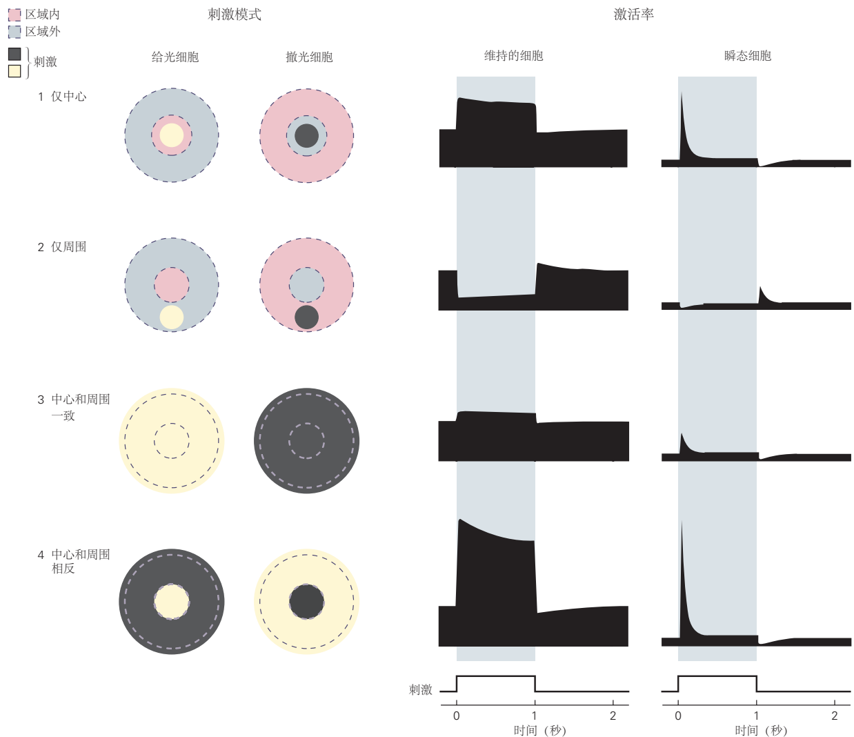
图 22.3.1: 具有中心环绕感受野的视网膜神经节细胞响应。在这些理想化的实验中，刺激从均匀的灰色区域变为左侧指示的明亮（黄色）和黑暗（黑色）区域的模式。这导致右侧显示的激活率响应。1. 给光细胞被感受野中心的亮点激发，撤光细胞被暗点激发。在持续细胞中，兴奋在整个刺激过程中持续存在，而在瞬态细胞中，在刺激开始后会出现短暂的脉冲。2. 如果将激发中心的相同刺激施加到周围，则会抑制放电。3. 中心和周围的均匀刺激引起与中心类似的响应，但幅度小得多。4. 中心的刺激与周围的相反刺激相结合会产生最强的响应。
