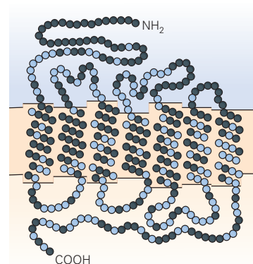
图 22.2.2: 视觉色素的结构。A. 视杆细胞中的视觉色素视紫红质是 2 种成分的共价复合物。视蛋白是一种大型蛋白质，具有 348 个氨基酸，分子量约为 4 万道尔顿。它在视杆细胞的膜上来回循环 7 次。视黄醛是一种小的吸光化合物，共价连接到视蛋白第 7 个跨膜区域赖氨酸 296 的侧链上。11-顺式视黄醛对光的吸收导致围绕双键的旋转。由于视网膜采用更稳定的全反式构型，它会引起视蛋白的构象变化，从而触发后续的视觉转导事件 [197] 。B. 蓝色圆圈表示相同的氨基酸；黑色圆圈表示差异。3 种视锥细胞（长波、中波和短波中的视蛋白形式彼此相似，视杆细胞中的视紫红质也相似，这表明这 4 种细胞都是通过复制和发散从一个共同的前体进化而来的。长波和中波视蛋白的关系最为密切，其氨基酸序列具有 96% 的同一性。它们被认为是从大约 3 千万年前的一次基因复制事件中进化而来的，当时旧大陆猴具有 3 种视觉色素，而新大陆猴通常只有 2 种。
