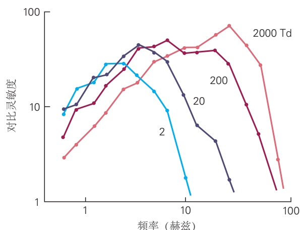
图 22.4.2: 时间对比敏感度。A. 人类受试者对时间闪烁的敏感性是通过类似于图 22.5.3A 中的方法测量的，但刺激是一个大点，其强度随时间呈正弦曲线变化，而不是在空间中。检测所需的阈值对比度的倒数相对于正弦闪烁的频率绘制。灵敏度在高频和低频均下降。平均光照水平发生变化，从顶部到底部轨迹减少了 10 倍。B. 猕猴视网膜中中波型神经节细胞的闪烁敏感性通过 A 部分中应用于人类受试者的相同方法测量。神经响应的检测阈值被定义为与闪烁同步的细胞发放率每秒 20 个脉冲的变化。
