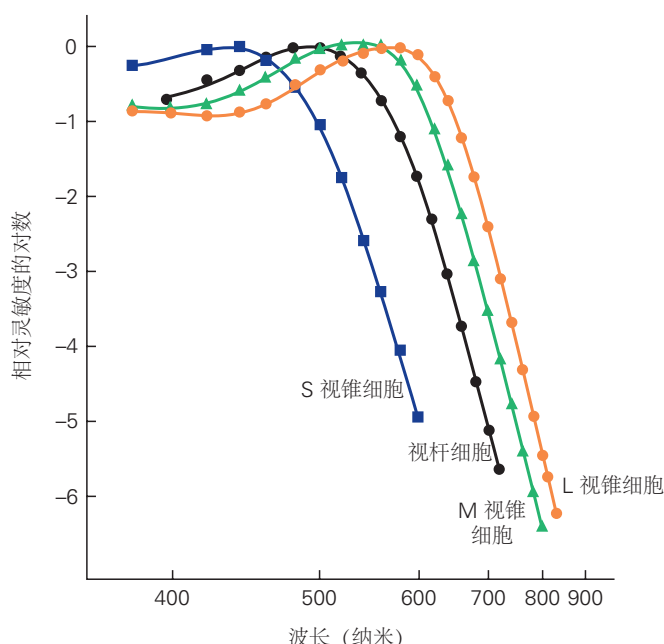
图 22.2.3: 3 种视锥细胞和视杆细胞的灵敏度光谱。在每个波长下，灵敏度与在感觉神经元中引起标准响应所需的光强度成反比。灵敏度在很大范围内变化，因此以对数刻度显示。不同类别的光受体对广泛且重叠的波长范围敏感。
