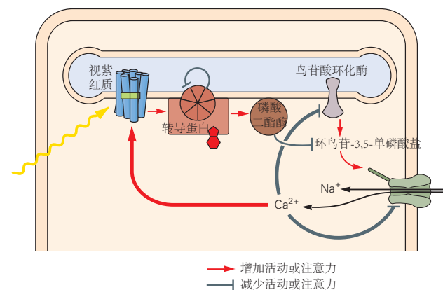
图 22.2.1: 光转导。 A. 视杆细胞对光有响应。外段视盘中的视紫红质分子吸收光子，导致细胞质膜中环鸟苷-3',5'-单磷酸盐门控通道关闭。这种通道关闭使膜超极化并降低神经递质谷氨酸的释放速率 [7] 。 B. 1. 光转导中的分子过程。环鸟苷-3',5'-单磷酸盐由鸟苷酸环化酶从三磷酸鸟苷产生并被磷酸二酯酶水解。在黑暗中，磷酸二酯酶活性低，环鸟苷-3',5'-单磷酸盐浓度高，环鸟苷-3',5'-单磷酸盐门控通道开放，允许 Na + 和 Ca 2+ 流入。在光线下，视紫红质通过吸收光子而被激发，然后激活转导蛋白，转导蛋白进而激活磷酸二酯酶；环鸟苷-3',5'-单磷酸盐水平下降，膜通道关闭，更少的 Na + 和 Ca 2+ 进入细胞。转导酶均位于内膜圆盘中，可溶性配体环鸟苷-3',5'-单磷酸盐作为细胞质膜的信使。 2. Ca 2+ 在光转导响应级联中具有负反馈作用。光对网络的刺激导致环鸟苷-3',5'-单磷酸盐门控通道的关闭。这导致细胞内 Ca 2+ 浓度下降。因为 Ca 2+ 调节至少 3 个级联组分的功能（视紫红质、鸟苷酸环化酶和环鸟苷-3',5'-单磷酸盐门控通道）Ca 2+ 的下降抵消了光引起的激发。 C. 灵长类视杆细胞和视锥细胞对强度增加的短暂闪光的电压响应。迹线上的数字越高表示光照强度越大（并非所有迹线都已标记）。对于昏暗的闪光，响应幅度随强度线性增加。在高强度下，受体饱和并在闪光后的一段时间内稳定地保持超极化；这会导致我们在明亮的闪光后看到的残像。请注意，对于更亮的闪光，响应峰值更早，并且视锥细胞的响应速度比视杆细胞快 [196] 。
