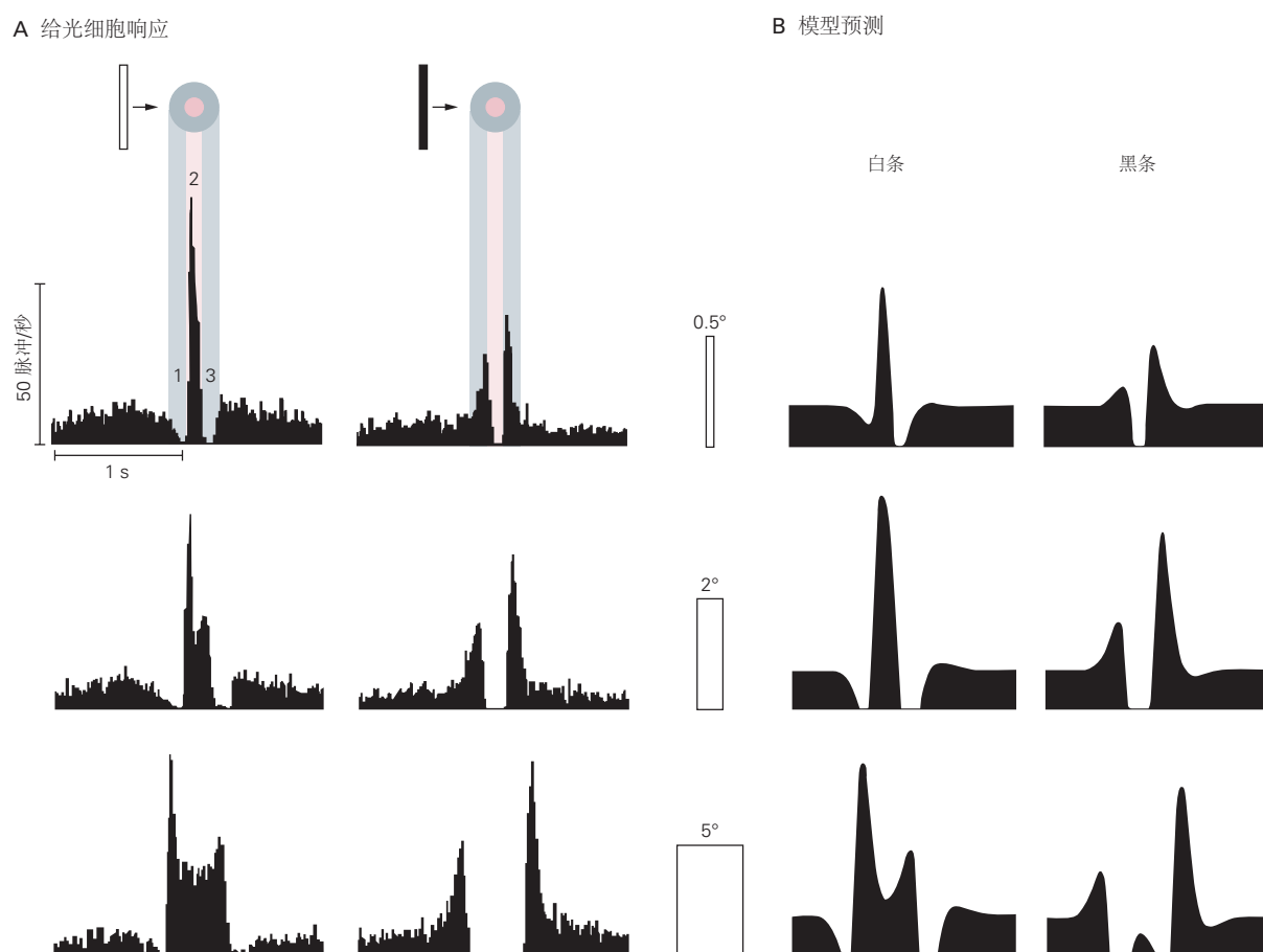
图 22.3.2: 猫视网膜神经节细胞对移动物体的响应。A. 给光神经节对各种横条（白色或黑色，不同宽度）在视网膜上移动的响应率。每个条以每秒 10^\circ 的速度移动； 1^\circ 对应于视网膜上的 180 微米。作为对白色条的响应，当条穿过感受野周围（1）时，激活率首先降低，随着条进入中心（2）而增加，当条形图穿过另一侧的周围时，激活率再次降低（3）。深色条引起相反符号的响应。由于与此类似的神经节细胞分布在整个视网膜中，因此也可以将此曲线解释为神经节细胞群活动的瞬时快照，其中横轴表示在视网膜上的位置。实际上，此激活概况是传输到大脑的移动条的神经表征。一个互补的撤光神经节细胞群（此处未显示）并行传达另一个神经活动概况。这样，亮边和暗边都可以通过激活的急剧增加来表示。B. 一个简单的视网膜处理模型，结合了中心环绕拮抗作用和瞬态时间过滤器，用于预测神经节细胞放电率。这些预测与 A 部分中响应的基本特征相匹配。
