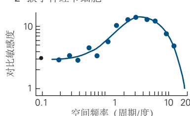
图 22.5.3: 空间对比敏感度。A. 1. 如图 22.5.4 所示，人类受试者的对比敏感度使用具有不同空间频率的光栅测量。如图所示，在每个频率下，对比度增加到检测阈值，并且该对比度值的倒数相对于空间频率绘制。这些曲线是在不同的平均强度下获得的，从顶部到底部曲线减少了 10 倍 [202] 。2. 在高强度下测量的猕猴视网膜中 P 型神经节细胞的对比敏感度。在每个空间频率下，对比度逐渐增加，直到它在神经元的放电率中产生可检测的变化。如 A-1 部分所示，绘制了该阈值对比度的倒数。左侧的孤立点标记了零空间频率下的灵敏度，这是一个空间均匀的场 [203] 。B. 用正弦光栅刺激中心环绕感受野。神经元对视网膜上不同点的光的敏感性被建模为“高斯差分”感受野，其中兴奋性中心为窄正高斯分布，抑制性周围为宽的负高斯分布。将光栅刺激的轮廓（强度与位置）与感受野的轮廓（灵敏度与位置）相乘，并在所有空间上积分，计算出特定光栅传递的刺激强度。右图显示了感受野对不同频率光栅的灵敏度。在低空间频率下，环绕声的负贡献抵消了中心的贡献，导致差异曲线下降 [204] 。
