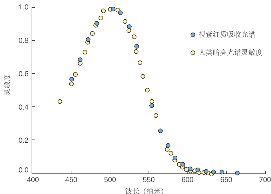
图 22.2.4: 视紫红质的吸收光谱。将在试管中测量的人类视紫红质的吸收光谱与人类观察者对非常暗淡的闪光的光谱灵敏度进行比较。心理物理数据已针对眼部介质的吸收进行了校正。
