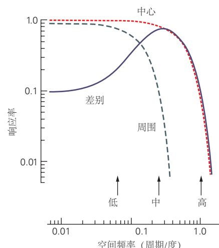
图 22.5.3: 空间对比敏感度。A. 1. 如图 22.5.4 所示，人类受试者的对比敏感度使用具有不同空间频率的光栅测量。如图所示，在每个频率下，对比度增加到检测阈值，并且该对比度值的倒数相对于空间频率绘制。这些曲线是在不同的平均强度下获得的，从顶部到底部曲线减少了 10 倍 [202] 。2. 在高强度下测量的猕猴视网膜中 P 型神经节细胞的对比敏感度。在每个空间频率下，对比度逐渐增加，直到它在神经元的放电率中产生可检测的变化。如 A-1 部分所示，绘制了该阈值对比度的倒数。左侧的孤立点标记了零空间频率下的灵敏度，这是一个空间均匀的场 [203] 。B. 用正弦光栅刺激中心环绕感受野。神经元对视网膜上不同点的光的敏感性被建模为“高斯差分”感受野，其中兴奋性中心为窄正高斯分布，抑制性周围为宽的负高斯分布。将光栅刺激的轮廓（强度与位置）与感受野的轮廓（灵敏度与位置）相乘，并在所有空间上积分，计算出特定光栅传递的刺激强度。右图显示了感受野对不同频率光栅的灵敏度。在低空间频率下，环绕声的负贡献抵消了中心的贡献，导致差异曲线下降 [204] 。
