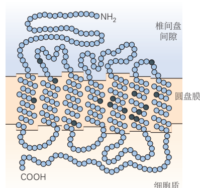
图 22.2.2: 视觉色素的结构。A. 视杆细胞中的视觉色素视紫红质是 2 种成分的共价复合物。视蛋白是一种大型蛋白质，具有 348 个氨基酸，分子量约为 4 万道尔顿。它在视杆细胞的膜上来回循环 7 次。视黄醛是一种小的吸光化合物，共价连接到视蛋白第 7 个跨膜区域赖氨酸 296 的侧链上。11-顺式视黄醛对光的吸收导致围绕双键的旋转。由于视网膜采用更稳定的全反式构型，它会引起视蛋白的构象变化，从而触发后续的视觉转导事件 [197] 。B. 蓝色圆圈表示相同的氨基酸；黑色圆圈表示差异。3 种视锥细胞（长波、中波和短波中的视蛋白形式彼此相似，视杆细胞中的视紫红质也相似，这表明这 4 种细胞都是通过复制和发散从一个共同的前体进化而来的。长波和中波视蛋白的关系最为密切，其氨基酸序列具有 96% 的同一性。它们被认为是从大约 3 千万年前的一次基因复制事件中进化而来的，当时旧大陆猴具有 3 种视觉色素，而新大陆猴通常只有 2 种。
