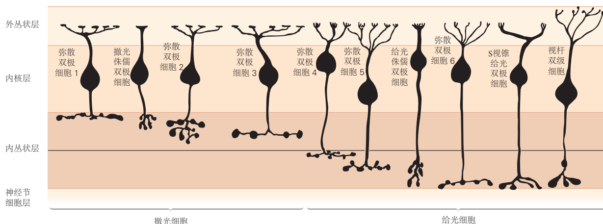
图 22.4.1: 猕猴视网膜中的双极细胞。细胞根据其在内网层中的末端分枝的深度排列。划分该层的远端（上）和近端（下）水平的水平线表示撤光型细胞和给光型细胞的轴突末梢之间的边界。假定上半部分的端子是撤光细胞的端子，下半部分的端子是给光单元的端子。细胞类型是弥散双极细胞、给光小型双极细胞和撤光小型双极细胞、短波锥双极细胞和杆状双极细胞。
