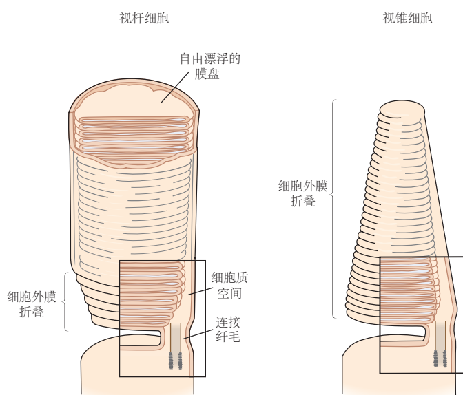
图 22.1.2: 视杆光受体和视锥光感受器具有相似的结构。A. 视杆细胞和视锥细胞都有称为外段和内段的特殊区域。外段通过纤毛连接到内段并包含光转换装置。内部部分包含线粒体和许多蛋白质合成机器。B. 外段由一堆含有吸光感光色素的膜盘组成。在这 2 种类型的细胞中，这些圆盘都是通过细胞质膜的折叠形成。然而，在杆状细胞中，褶皱从膜上夹断，因此圆盘在外段内自由漂浮，而在视锥细胞中，圆盘仍然是细胞质膜的一部分 [194-195] 。
