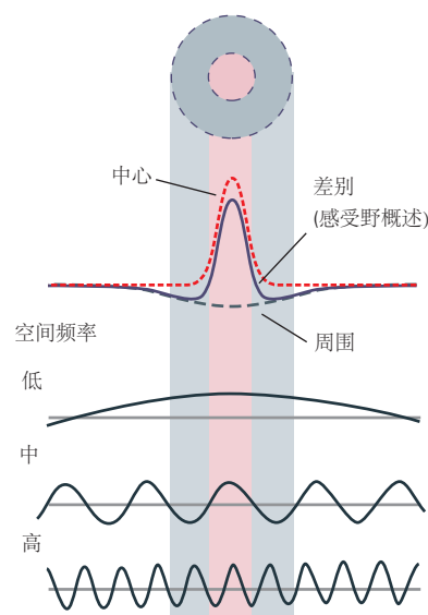
图 22.5.3: 空间对比敏感度。A. 1. 如图 22.5.4 所示，人类受试者的对比敏感度使用具有不同空间频率的光栅测量。如图所示，在每个频率下，对比度增加到检测阈值，并且该对比度值的倒数相对于空间频率绘制。这些曲线是在不同的平均强度下获得的，从顶部到底部曲线减少了 10 倍 [202] 。2. 在高强度下测量的猕猴视网膜中 P 型神经节细胞的对比敏感度。在每个空间频率下，对比度逐渐增加，直到它在神经元的放电率中产生可检测的变化。如 A-1 部分所示，绘制了该阈值对比度的倒数。左侧的孤立点标记了零空间频率下的灵敏度，这是一个空间均匀的场 [203] 。B. 用正弦光栅刺激中心环绕感受野。神经元对视网膜上不同点的光的敏感性被建模为“高斯差分”感受野，其中兴奋性中心为窄正高斯分布，抑制性周围为宽的负高斯分布。将光栅刺激的轮廓（强度与位置）与感受野的轮廓（灵敏度与位置）相乘，并在所有空间上积分，计算出特定光栅传递的刺激强度。右图显示了感受野对不同频率光栅的灵敏度。在低空间频率下，环绕声的负贡献抵消了中心的贡献，导致差异曲线下降 [204] 。
