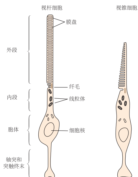
图 22.1.2: 视杆光受体和视锥光感受器具有相似的结构。A. 视杆细胞和视锥细胞都有称为外段和内段的特殊区域。外段通过纤毛连接到内段并包含光转换装置。内部部分包含线粒体和许多蛋白质合成机器。B. 外段由一堆含有吸光感光色素的膜盘组成。在这 2 种类型的细胞中，这些圆盘都是通过细胞质膜的折叠形成。然而，在杆状细胞中，褶皱从膜上夹断，因此圆盘在外段内自由漂浮，而在视锥细胞中，圆盘仍然是细胞质膜的一部分 [194-195] 。
