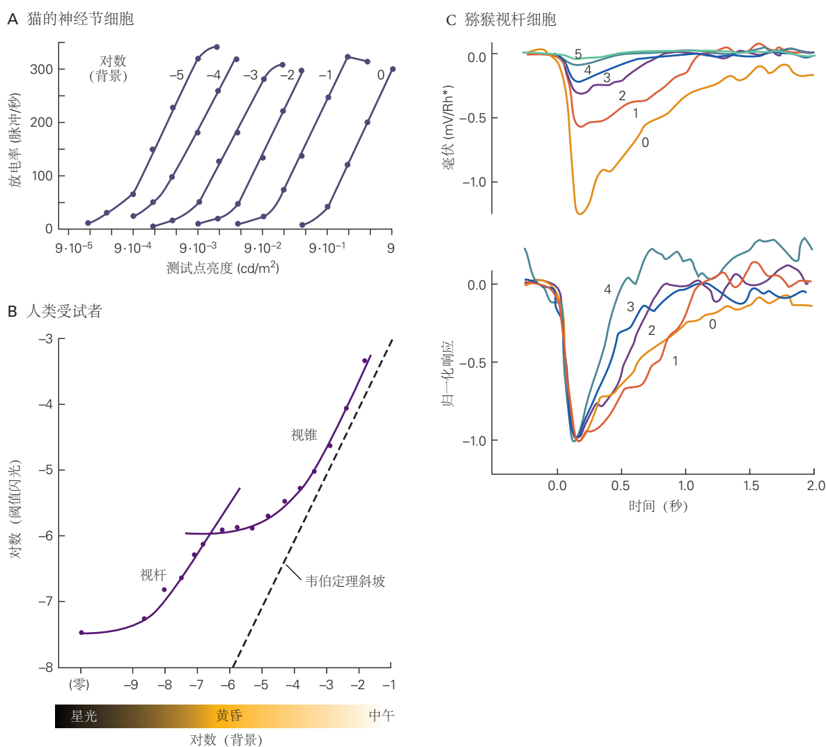
图 22.5.2: 光照适应。 A. 猫视网膜神经节细胞的感受野在稳定的背景强度下均匀照明, 并在感受野中心短暂闪烁一个测试点。测量闪光后的峰值激活率并根据闪光强度的对数绘制。每条曲线对应不同的背景强度, 从左到右增加 10 倍 [199] 。B. 一个小的测试点在稳定照明的背景上短暂闪光, 闪光强度逐渐增加到人类受试者刚好可以检测到的程度。在不同的背景强度下重复该过程。这里, 阈值闪光强度根据背景强度绘制。该曲线有 2 个分支, 由一个明显的扭结相连: 它们对应于视杆视觉和视锥视觉的状态。当阈值强度与背景强度成正比时, 韦伯定律的斜率表示理想化 [200] 。C. 上图显示了猕猴视杆细胞对不同背景强度下出现闪光的响应。细胞的单光子响应根据记录的膜电位除以闪光激活的视紫红质的数量计算得出。单光子响应的增益随着背景强度的增加而显著降低。背景强度 (以光子/平方微米/秒为单位) 对于迹线 0 为 0, 对于迹线 1 为 3.1, 对于迹线 2 为 12, 对于迹线 3 为 41, 对于迹线 4 为 84, 对于迹线 5 为 162。在底部图中, 相同数据 (最小响应除外) 被归一化为相同的振幅, 表明单光子响应的时间进程在高强度下加速 [201] 。
