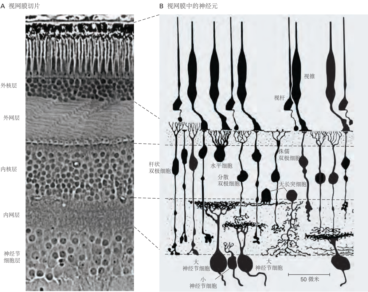
图 22.0.2: 视网膜包括 5 个不同的神经元和突触层。A. 通过光学显微镜看到的人类视网膜的垂直截面。3 层细胞体明显。外核层包含感光细胞体；内核层包括水平细胞、双极细胞和无长突细胞；神经节细胞层含有神经节细胞和一些移位的无长突细胞。2 层纤维和突触将它们分开：外网层和内网层 [191] 。B. 基于高尔基体染色的猕猴视网膜神经元。细胞层和突触层与 A 部分中的图像对齐 [192] 。
