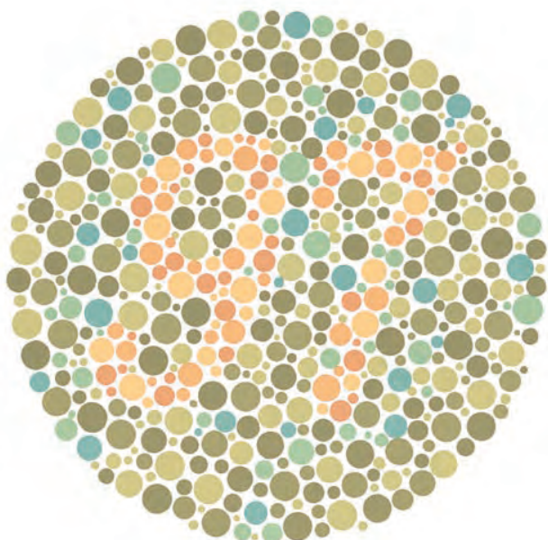
图 22.4.3: 对某些形式的色盲测试。嵌入这种颜色图案中的数字可以被具有三色视觉的人辨别出来，但不能被红绿辨别力较弱的二色视者辨别出来。如果您没有看到任何数字，请检查您的视力。
