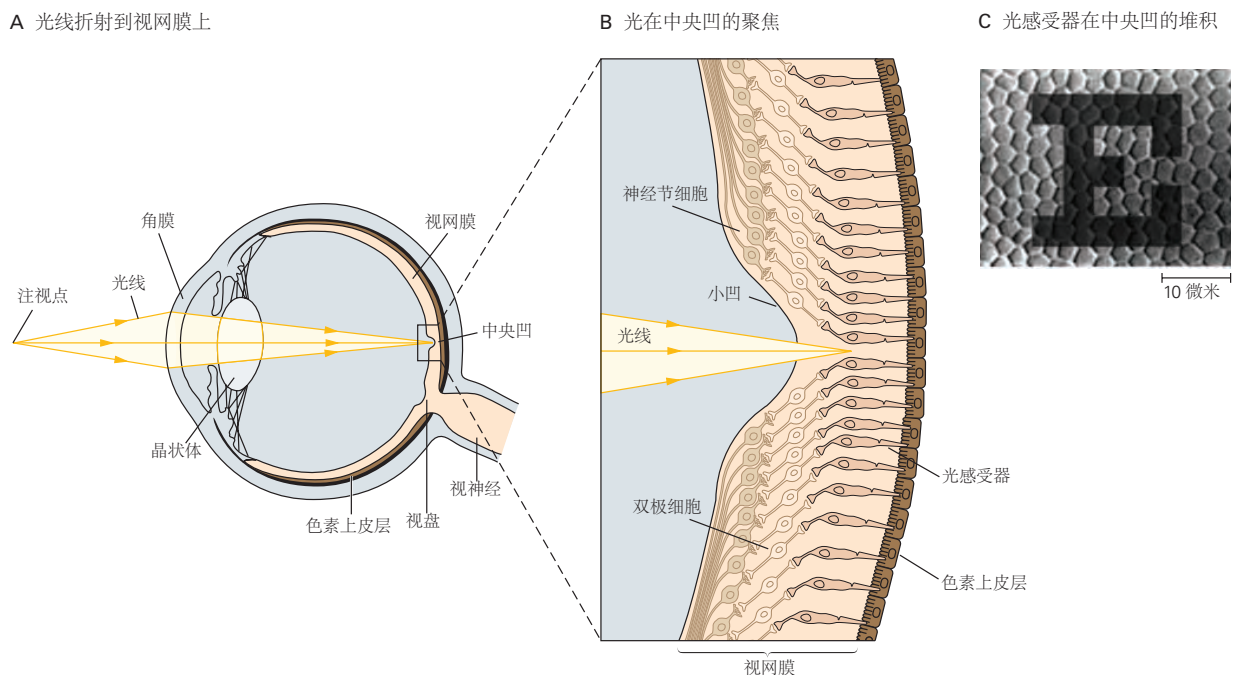
图 22.0.1: 眼睛将视觉场景投射到视网膜的感光器上。A. 来自视野中物体的光被角膜和晶状体折射并聚焦到视网膜上。B. 在中央凹，对应于凝视的正中心，视网膜的近端神经元被移到一边，因此光线可以直接进入光受体。C. 用于评估正常视力的视力表中的字母被投射到中央凹中密集的光受体上。由于肉眼的光学衍射，虽然不像这里显示的那样清晰，但字母的最小可辨别笔画宽度约为一个视锥细胞直径 [190] 。
