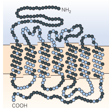
图 22.2.2: 视觉色素的结构。A. 视杆细胞中的视觉色素视紫红质是 2 种成分的共价复合物。视蛋白是一种大型蛋白质，具有 348 个氨基酸，分子量约为 4 万道尔顿。它在视杆细胞的膜上来回循环 7 次。视黄醛是一种小的吸光化合物，共价连接到视蛋白第 7 个跨膜区域赖氨酸 296 的侧链上。11-顺式视黄醛对光的吸收导致围绕双键的旋转。由于视网膜采用更稳定的全反式构型，它会引起视蛋白的构象变化，从而触发后续的视觉转导事件 [197] 。B. 蓝色圆圈表示相同的氨基酸；黑色圆圈表示差异。3 种视锥细胞（长波、中波和短波中的视蛋白形式彼此相似，视杆细胞中的视紫红质也相似，这表明这 4 种细胞都是通过复制和发散从一个共同的前体进化而来的。长波和中波视蛋白的关系最为密切，其氨基酸序列具有 96% 的同一性。它们被认为是从大约 3 千万年前的一次基因复制事件中进化而来的，当时旧大陆猴具有 3 种视觉色素，而新大陆猴通常只有 2 种。
