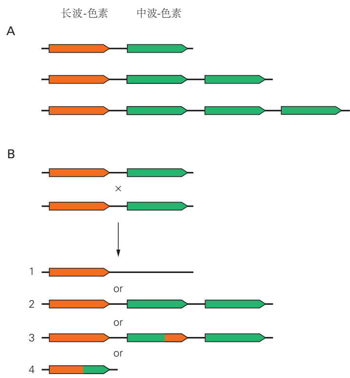
图 22.4.4: X 染色体上的长波和中波色素基因。A. 长波-色素基因和中波-色素基因通常在染色体上彼此相邻。每个箭头的底部对应基因的 5' 端，尖端对应基因的 3' 端。具有正常色觉的男性在每条 X 染色体上可能有 1 个、2 个或 3 个中波色素基因拷贝 [198] 。B. 长波-色素基因和中波-色素基因的重组可导致杂合基因 (3 和 4) 的产生或丢失基因 (1) 的模式，在色盲男性中观察到的模式。虚假重组也可能导致基因复制 (2)，这是在一些具有正常色觉的人身上观察到的模式。
