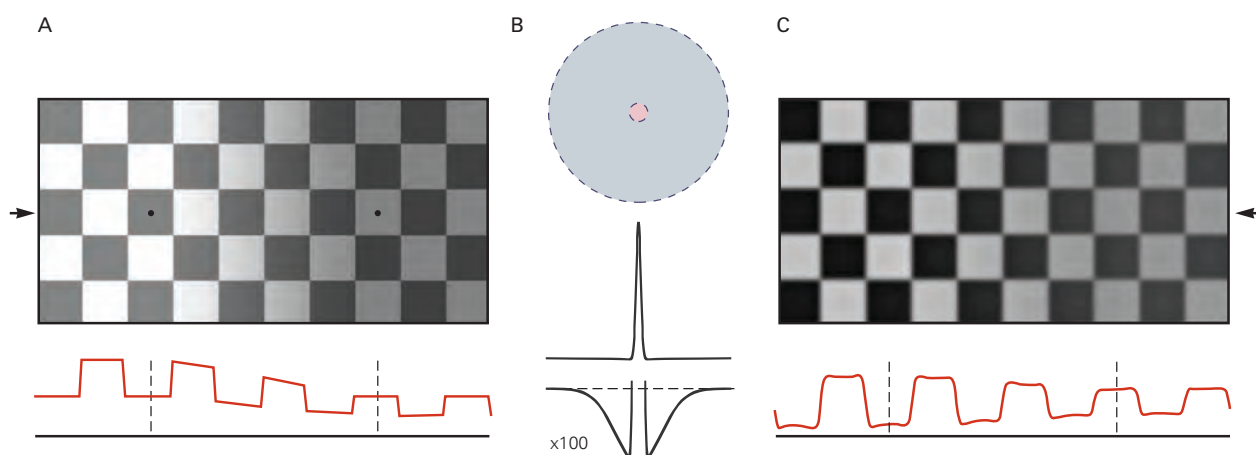
图 22.5.1: 亮度错觉。 A. 标有小点的 2 块瓷砖看起来颜色不同，但实际上反射的光强度相同（要看到这一点，请折叠页面，使它们接触）。下方的迹线绘制了箭头水平的光强度分布图。您的视觉系统将此视网膜图像解释为空间变化照明下的规则图块图案，右半部分有漫射阴影。根据这种解释，右边的瓷砖必须比左边的颜色浅，这就是您所感知的。这个过程是自动的，不需要有意识的分析。B. 视网膜处理通过降低阴影平滑的照明梯度并突出棋盘区域之间的锐利边缘来促进“亮度”的感知。具有兴奋中心和抑制周围的视觉神经元的感受野显示在顶部。如底部放大百倍所示，环绕声较弱，但延伸的区域比中心区域大得多。C. 当一群具有 B 中感受野的视觉神经元处理 A 中的图像时的结果。这个操作（A 中的图像与 B 中的轮廓的卷积）从视野中的每个点中减去大周围区域的平均强度。目标的神经表示在很大程度上失去了阴影的影响，并且所讨论的 2 个图块在该表示中确实具有不同的亮度值。
