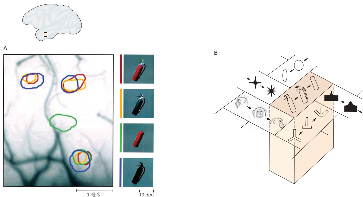
图 24.2.4: 下颞皮层前部对复杂视觉刺激作出响应的神经元被组织成柱。A. 前下颞皮层表面的光学图像说明了被右侧所示目标选择性激活的区域。B. 下颞皮层的神经元组织成从皮层表面延伸出来的功能特化柱。根据这个模型，每一柱都包含对特定视觉复杂目标做出响应的神经元。代表一个目标变化的神经元柱（例如不同的面孔或不同的激活灭火器）构成了一个皮层柱。
