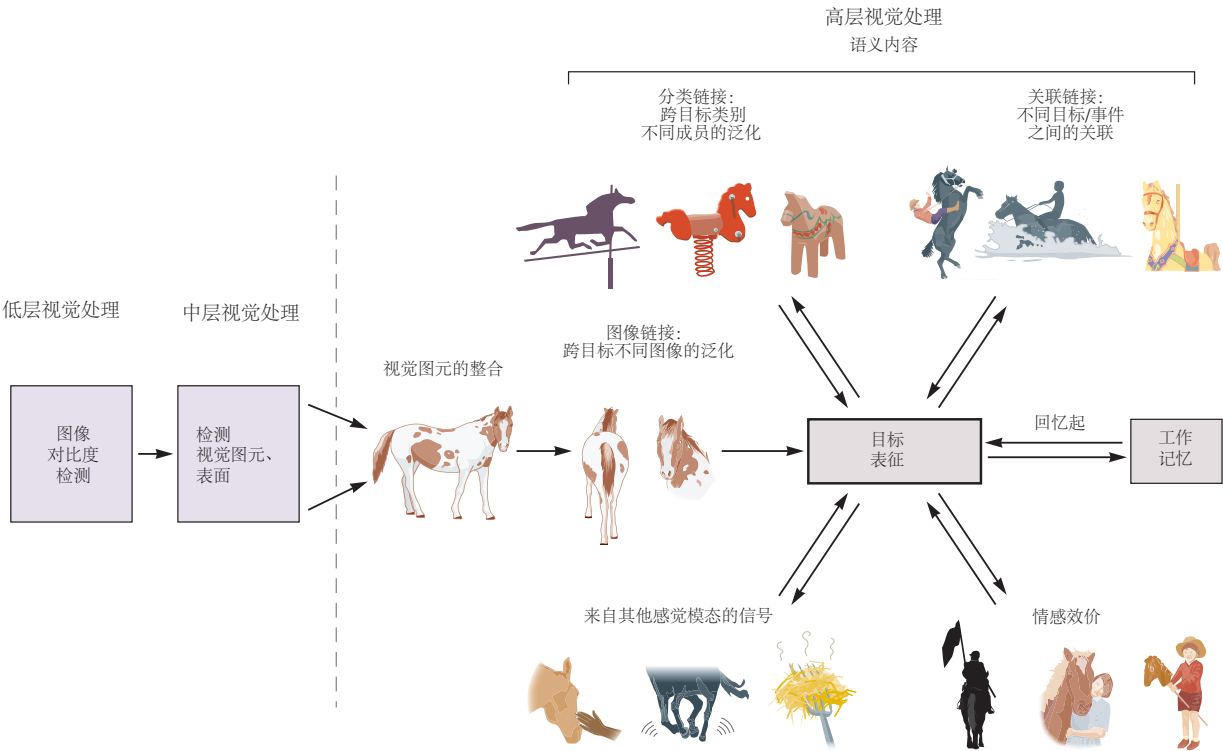
图 24.1.1: 整个目标的表示是高层视觉处理的核心。整个目标的表示涉及视觉通路的早期阶段提取视觉特征的整合。这种整合是由同一目标和目标类别的不同成员生成大量视网膜图像概括。该表示还结合了来自其他感官模态的信息（附加情感效价），并将该目标与其他目标或事件的记忆相关联。目标表示可以存储在工作记忆中，并与其他记忆相关联而回忆起来。
