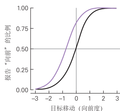
图 25.1.5: 感知到的眼跳方向随着伴随发送的中断而改变。A. 在每次试验开始时，猴子都会在屏幕上注视一个目标 (1)。当注视点关闭时，猴子会向目标眼跳；在眼跳期间，目标随机 (最多 3^\circ ) 向左或向右移动 (2)。在眼跳到原始目标后，猴子会收到一个奖励，用于在目标位移的方向上手动移动一个杆 (3)。B. 丘脑内侧背核失活之前 (黑色) 和失活之后 (紫色) 的心理测量曲线，其中包含在上丘和额叶皮层之间的通路中进行伴随发送的中继神经元。该曲线显示了每个目标位移 (x 轴) 的向前 (在眼跳方向) 判断 (y 轴) 的比例。猴子没有感知到位移的眼跳后目标位置被定义为感知零点 [226] 。
