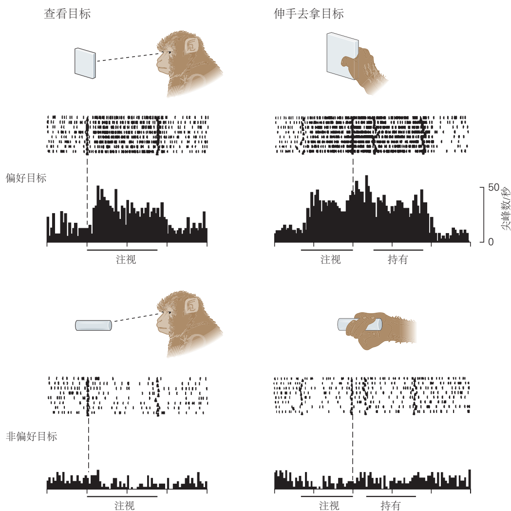
图 25.3.2: 顶内前皮层的神经元对特定的形状有选择性的响应。这里显示的神经元对矩形是有选择性的，无论是观察物体还是伸手去够。无论哪种情况，神经元都对圆柱体没有响应。
