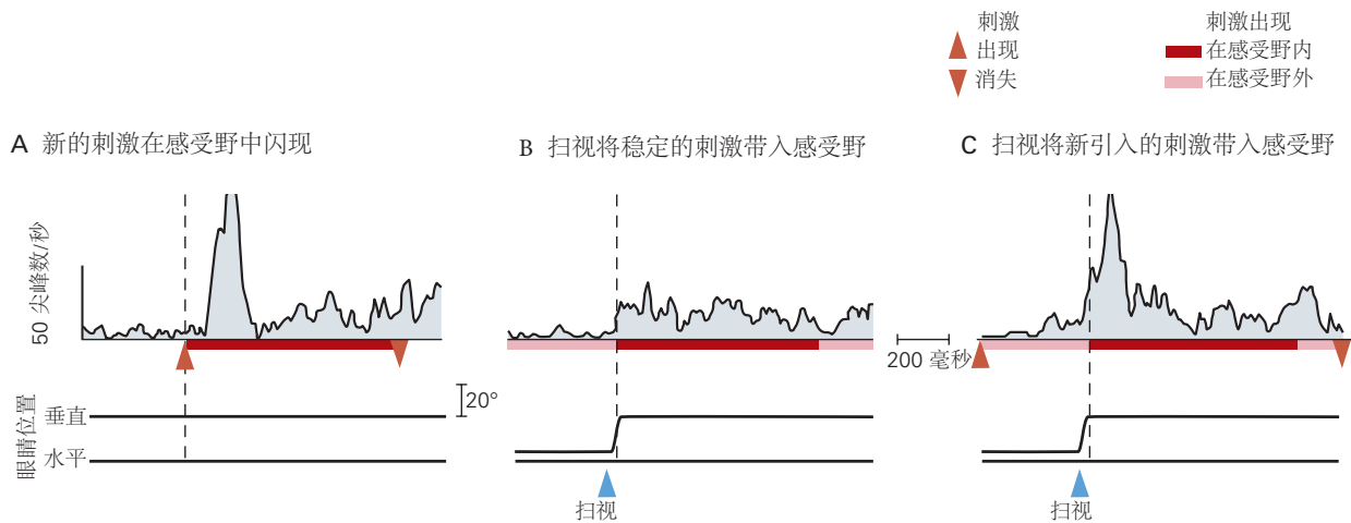
图 25.2.4: 顶内外侧区域的神经元仅在对显著刺激做出响应时才会放电。在每个面板中，神经元活动和眼睛位置都是随时间绘制的。A. 猴子注视时，感受野中会闪现一个刺激。B. 猴子的眼跳将稳定的、与任务无关的刺激带入感受野。C. 猴子做一个眼跳动作，将最近闪光的位置带入感受野。
