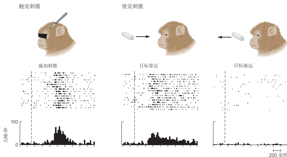
图 25.3.3: 猴子顶内皮层腹侧的双模态神经元对视觉和触觉刺激都有响应。这里显示的神经元对猴子头部的触觉刺激或朝向头部的视觉刺激做出响应，但对远离头部的相同刺激没有响应。
