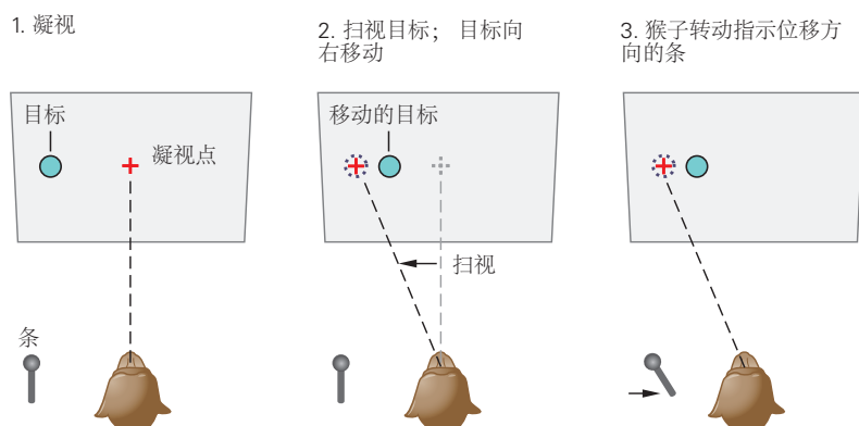
图 25.1.5: 感知到的眼跳方向随着伴随发送的中断而改变。A. 在每次试验开始时，猴子都会在屏幕上注视一个目标 (1)。当注视点关闭时，猴子会向目标眼跳；在眼跳期间，目标随机 (最多 3^\circ ) 向左或向右移动 (2)。在眼跳到原始目标后，猴子会收到一个奖励，用于在目标位移的方向上手动移动一个杆 (3)。B. 丘脑内侧背核失活之前 (黑色) 和失活之后 (紫色) 的心理测量曲线，其中包含在上丘和额叶皮层之间的通路中进行伴随发送的中继神经元。该曲线显示了每个目标位移 (x 轴) 的向前 (在眼跳方向) 判断 (y 轴) 的比例。猴子没有感知到位移的眼跳后目标位置被定义为感知零点 [226] 。
