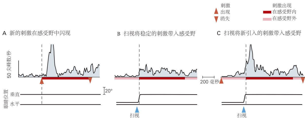
图 25.2.5: 在眼跳一个重要的稳定物体之前，位于顶内外侧区域的神经元会启动。在每次试验中，稳定阵列中的一个物体对猴子来说都很重要，因为猴子必须对它进行眼跳。猴子注视阵列外的一个点，与阵列中的物体匹配的线索出现在神经元的感受野外。然后，猴子必须眼跳阵列的中心，再扫视与线索匹配的物体。显示了 2 个实验（在 A 和 B 部分中）。左侧面板显示神经元对感受野外提示出现的响应，中间面板显示第一次眼跳将提示目标带入感受野后的响应，右侧面板显示第二次扫视前对提示对象的响应。为了清晰起见，这里的提示是绿色的，但在实验中是黑色的。在 2 个实验中，眼跳时的视觉场景是相同的。A. 训练猴子对提示的物体进行第二次眼跳；当第一次眼跳将物体带入感受野时，细胞会强烈地激发。B. 训练猴子对感受野外的物体进行第二次眼跳；当眼跳将与任务无关的刺激带入感受野时，细胞激发的能量要少得多。
