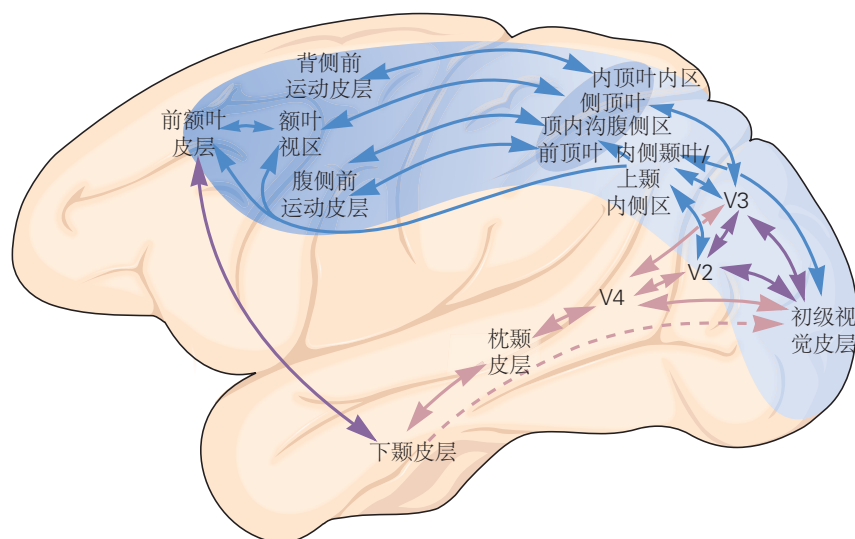
图 25.3.1: 动作视觉处理的通路。背侧视觉通路（蓝色）延伸到后顶叶皮层，然后延伸到额叶皮层。腹侧视觉通路（粉红色）见第 24 章。从下颞皮层到前额叶皮层有双向投射。
