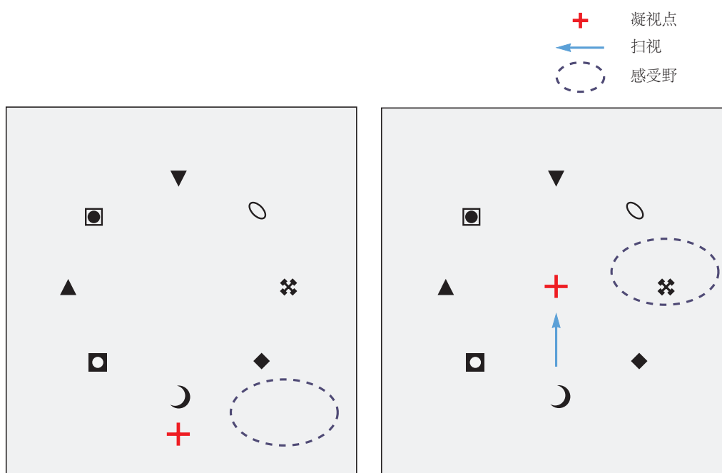
图 25.2.3: 探索一组稳定的物体。猴子观看一个屏幕，屏幕上有许多物体在整个实验过程中都保持不变。猴子的凝视可以定位为使任何物体都不包括在神经元的感受野中（左），或者猴子可以进行眼跳，将其中一个物体带入感受野（右）。
