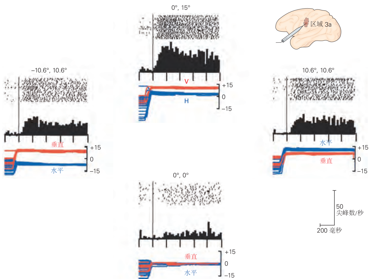
图 25.1.7: 体感皮层区 3a 中的眼睛位置神经元。每个面板显示水平和垂直眼睛位置以及猴子对每个光栅上方指示的眼睛位置进行眼跳后神经元的活动。当眼睛处于 0^\circ, 15^\circ 时，神经元的响应比在 0^\circ, 0^\circ 时要快得多。
