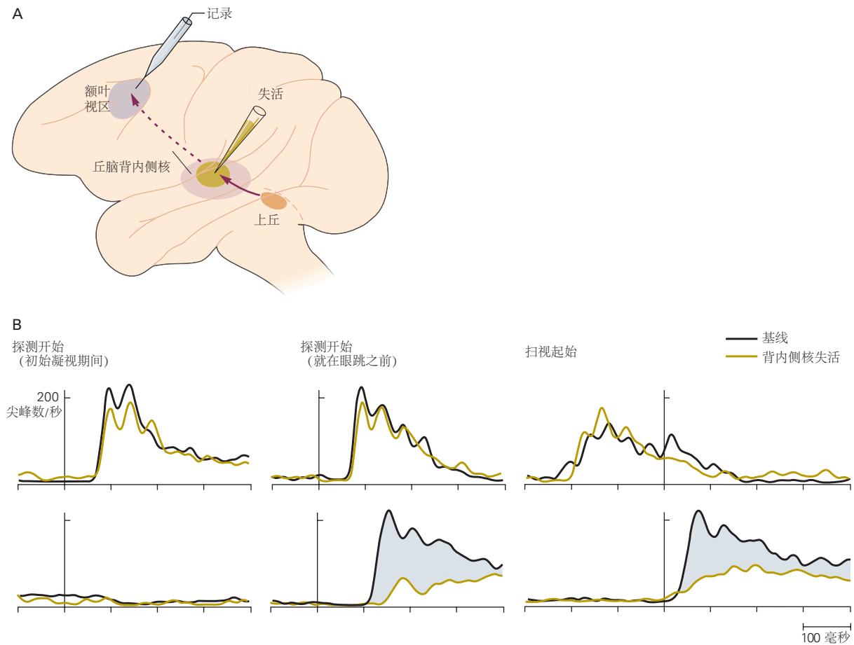
图 25.1.4: 来自眼跳运动程序的伴随发送会导致在扫视之前额叶视区神经元的感受野位置发生变化 [225] 。A. 伴随发送的一种可能通路起源于上丘中产生眼跳的神经元，穿过丘脑的内侧背核，并终止于额叶皮层的额叶视区。B. 当背内侧核失活时，额叶视区神经元对细胞当前感受野中刺激探针的响应不受影响（上部记录），而对未来刺激（后-眼跳）感受野严重受损（记录较低）。这一结果表明，眼跳运动程序的伴随发送指导神经元感受野特性的转变。
