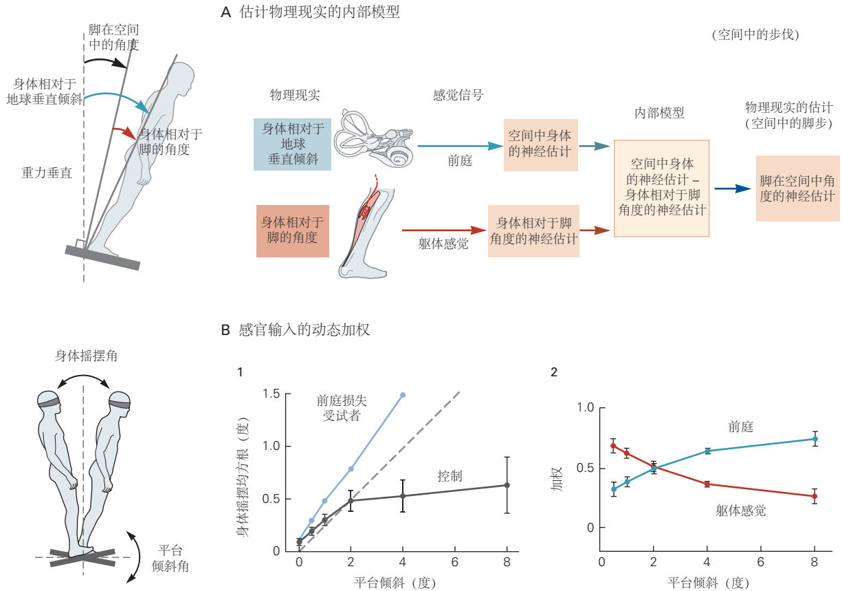
图 36.3.4: 许多类型的感官信号在优化平衡和方向的内部模型中被集成和加权 [358] 。A. 一个人站在倾斜的表面上简单的例子说明了神经系统如何估计无法直接感知的物理变量。物理变量是身体相对于地球垂直倾斜，以及身体相对于脚的角度。脚在空间中的角度就是差值身体相对于地球垂直倾斜 - 身体相对于脚的角度。空间中身体的神经估计来自前庭和其他检测身体相对于重力倾斜的受体。身体相对于脚角度的神经估计来自与踝关节角度相关的体感信号。用于估计物理现实的内部模型空间中身体的神经估计 - 身体相对于脚角度的神经估计产生脚在空间中角度的神经估计。这种对物理世界的估计会根据经验不断更新。B. 感官信息动态加权以在不同条件下保持平衡和定向。该图说明了一项实验的结果，在该实验中，人类受试者蒙着眼睛站在一个平台上，该平台以高达 8°（峰到峰）的幅度在脚趾向上或脚趾向下的方向上连续缓慢旋转。1. 前庭功能丧失的受试者和一组对照受试者在表面振荡期间身体摇摆的比较。车身摇摆角是在平台倾斜期间相对于重力垂直方向测量的，并表示为以度为单位的均方根摇摆。虚线代表平等的平台和身体摇摆；例如，对于 4° 的平台倾斜，等量的身体摇摆是 1° 均方根。在控制对象中，身体和平台的摇摆对于小平台倾斜高达 2° 是相等的，这表明人们通常使用体感信号来保持与平台的垂直（最小化脚踝角度的变化）。对于更大的平台倾斜度，车身摇摆不会增加太多超过 0.5° 均方根。相比之下，前庭功能丧失的受试者比平台摇摆得更多（平台倾斜度为 4° 时身体倾斜度为 1.5° 均方根）并且不能在平台倾斜度超过 4° 时保持站立。因此，当前庭信号和视觉信号均不存在时，人试图仅相对于支撑表面保持其位置并且难以在该表面移动时保持平衡。2. 在控制对象中，随着平台倾斜度的增加，体感输入的影响随着平台倾斜度的增加而减小，而前庭输入的影响增加。在更大的倾斜角度下，前庭输入的影响更大，可以最大限度地减少身体偏离重力垂直方向的程度。
