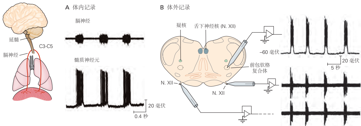
图 40.3.2: 在延髓内产生有节奏的呼吸。A. 豚鼠膈运动神经的节律活动导致横膈膜收缩。膈神经的放电被锁相到延髓中神经元的放电爆发。显示了细胞内记录的单个延髓神经元的活动 [380] 。B. 类似的节律性放电可以从副呼吸神经（例如舌下神经（XII））在体外记录到。支持这种节律所需的最小组织是延髓头端水平约 0.5 毫米厚的切片。前包钦格复合体中的神经元靠近与运动节律锁相的疑核激活爆发 [381] 。
