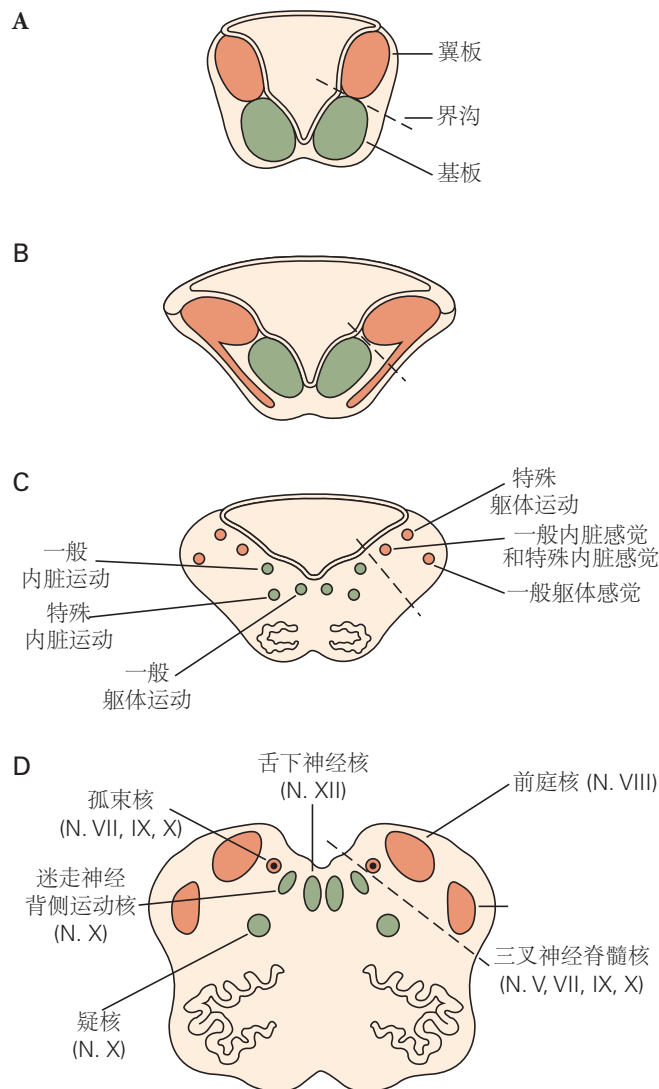
图 40.2.1: 脑干的发育计划与脊髓的总体计划相同。A. 神经管被纵沟、界沟分为背侧感觉部分（翼板）和腹侧运动部分（基底板）。B-D. 在发育过程中，感觉细胞群和运动细胞群迁移到它们成年的位置，但在很大程度上保留了它们的相对位置。在成熟期（D 部分），在第四脑室壁和脑导水管中仍可识别到界沟（虚线），划分了背侧感觉（橙色）和腹侧运动（绿色）结构之间的边界。D 部分的部分来自延髓嘴侧。
