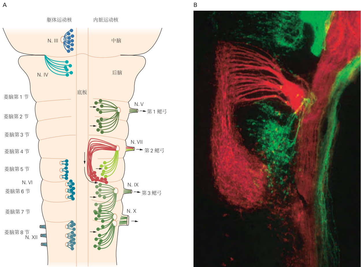
图 40.2.2: 胚胎颅神经核团是分段组织的。A. 在发育中的后脑（此处从腹侧看），除菱脑第 1 节外，每个后脑节段（菱脑节）都形成了特殊和一般的内脏运动神经元（代表在脑干的右侧）。每个特殊的内脏运动核由 2 个菱形神经元组成：三叉神经运动核由菱脑第 2 节和菱脑第 3 节神经元组成，面神经核由菱脑第 4 节和菱脑第 5 节神经元组成，舌咽核由菱脑第 6 节和菱脑第 7 节神经元组成，舌咽神经核由菱脑第 6 节和菱脑第 7 节神经元组成，由菱脑第 7 节和菱脑第 8 节中的神经元引起的迷走神经。这些核中每一个的神经元轴突在脑内横向走行，通过外侧神经上皮（菱脑第 2、4、6 和 7 节）的出口点离开大脑，并在脑外一起运行以形成各自的颅运动神经（V, VII, IX, X）。三叉神经（V）神经支配第 1 鳃弓的肌肉，面神经（VII）支配第 2 鳃弓的肌肉，舌咽（IX）神经支配第 3 鳃弓的肌肉。所有的内脏运动神经元（各种深浅不一的绿色，代表在脑干的右侧）最初在腹侧中线的底板旁边发育；在将它们的轴突延伸到它们各自的出口点后，细胞体然后横向迁移（箭头）。例外是在菱脑第 4 节（红色）中形成的面部运动神经元；细胞体在向出口点延伸其轴突后，在横向迁移之前向尾端迁移到菱脑第 6 节的轴向水平。与神经 VII（浅绿色）相关的一般内脏（副交感神经）运动神经元采取更传统的过程（见面板 B）。菱脑第 1 节（滑车核）、菱脑第 5 节和菱脑第 6 节（外展核）以及菱脑第 8 节（舌下核）形成了一般躯体运动核（各种深浅不一的蓝色，代表在脑干的左侧）。这些神经元的细胞体仍然靠近它们的出生地，即靠近底板。外展神经元和舌下神经元的轴突直接从腹侧离开大脑，没有横向走行。滑车神经元（浅蓝色）的轴突在脑内横向延伸和背侧延伸，直到下丘尾部向内侧转动，在下丘后面交叉，并在对侧中线附近退出。B. 小鼠胚胎的脑干，其中荧光染料标记了不同的颅神经 VII 运动神经元群。一种红色荧光染料通过来自面神经运动根的逆行运输填充面部运动神经元的细胞体。这些神经元最初在菱脑第 4 节中发育，然后沿着底板向后迁移到菱脑第 6 节（参见 A 部分中的红色神经元）。一种绿色荧光染料通过从中间神经根（感觉和神经节前一般内脏运动轴突）的逆行运输填充菱脑第 5 节中一般内脏运动神经元的细胞体（见 A 部分中的浅绿色神经元）。
