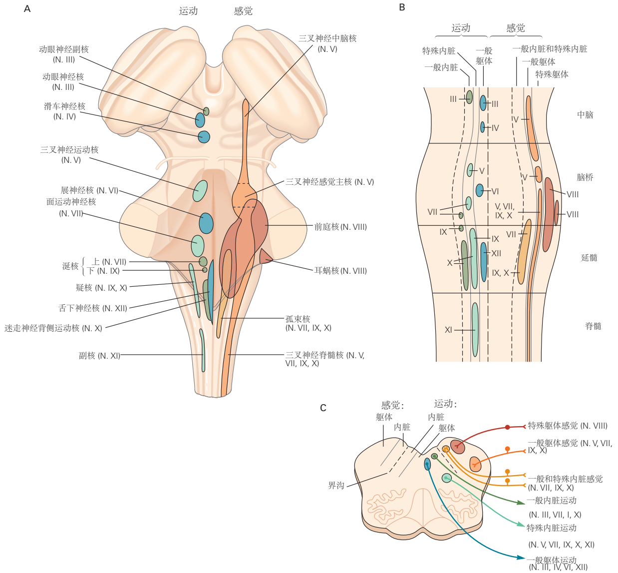
图 40.2.3: 成人颅神经核团在脑干的头尾轴上分为 6 个功能柱。A. 这张人的脑干背面图显示了颅神经感觉核 (右) 和运动核 (左) 的位置。B. 颅神经核团的功能组织示意图更清楚地表明它们形成运动柱和感觉柱。C. 与图 40.2.1D 比较, 颅神经核的内侧-外侧排列显示在延髓水平的横截面中。
