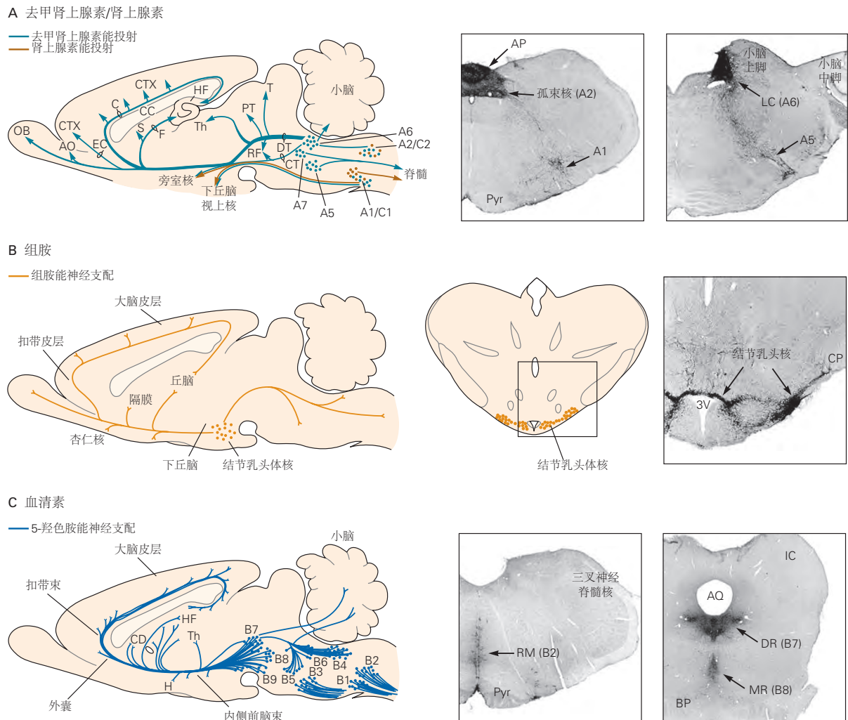
图 40.4.1: 大鼠大脑中单胺能和胆碱能神经元的位置和投射。A. 去甲肾上腺素能神经元 (A 组) 和肾上腺素能神经元 (C 组) 位于延髓和脑桥。延髓背侧的 A2 和 C2 组是孤束核的一部分。腹侧延髓中的 A1 和 C1 组位于疑核附近。2 组都投射到下丘脑; 一些 C1 神经元投射到脊髓中的交感神经节前神经元并控制心血管和内分泌功能。脑桥中的 A5、A6 (蓝斑) 和 A7 细胞群投射到脊髓并调节自主神经反射和痛觉。蓝斑也突出到前脑, 在唤醒和注意力方面起着重要作用。B. 所有组胺能神经元都位于下丘脑后外侧, 大部分位于结节乳头核内。这些神经元几乎投射到神经轴的每个部分, 并在唤醒中发挥重要作用。C. 5-羟色胺能神经元 (B 组) 存在于延髓、脑桥和中脑内, 大部分位于中缝核的中线附近。延髓内的那些 (对应于大中缝、不定中缝和苍白中缝的 B1-B4 组) 投射到整个延髓和脊髓并调节传入疼痛信号、体温调节、心血管控制和呼吸。脑桥和中脑内的那些 (脑桥中缝、中缝和中缝背侧的 B5-B9 组) 投射到整个前脑并有助于觉醒、情绪和认知。
