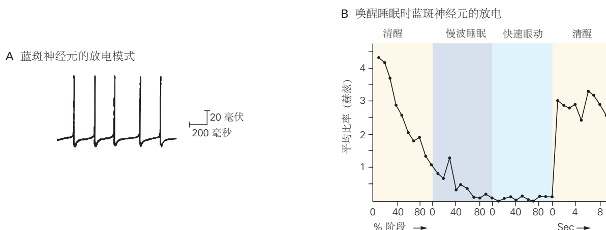
图 40.4.3: 单胺能神经元在整个觉醒-睡眠周期中具有相似的放电模式。A. 当单胺能神经元与突触输入隔离时，它们会以固定速率自发放电。这段记录来自蓝斑中的去甲肾上腺素能神经元。动作电位之后是特征性的后超极化，然后是下一个脉冲的缓慢去极化，产生类似起搏器的活动（第 10 章）。5-羟色氨酸能和组胺能神经元表现出相似的自发活动。B. 所有 3 种单胺能细胞类型在整个觉醒-睡眠周期中都显示出相似的激活模式。该图显示大鼠的蓝斑神经元在动物觉醒时放电最快，随着清醒减弱和慢波睡眠减慢，并且在睡觉快速眼动期间几乎完全停止放电 [386] 。
