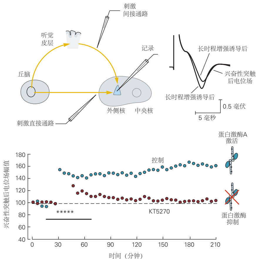
图 53.4.3: 杏仁核中突触的长时程增强可能会介导威胁条件反射。A. 小鼠的冠状脑切片显示了杏仁核的位置。放大图显示了杏仁核的 3 个关键输入核：外侧核、基底外侧核和基底内侧核，它们一起形成了基底外侧复合体。这些核投射到中央核，中央核投射到下丘脑和脑干 [507] 。B. 从丘脑到侧核的直接或间接通路的高频强直刺激启动长时程增强。该图显示了细胞外电压记录电极在侧核中的位置，以及用于激活直接通路或间接通路的 2 个刺激电极的位置。该图显示了在实验过程中细胞外兴奋性突触后电位场响应间接皮层通路刺激的振幅。当以低频率（每 30 秒一次）刺激通路时，兴奋性突触后电位场是稳定的。然而，当应用 5 列高频强直刺激（星号）时，响应会增强数小时。这种促进作用取决于蛋白激酶 A，并且在应用蛋白激酶 A 抑制剂 KT5720 时会受到影响（柱状图）。还显示了诱导长时程增强之前和之后的兴奋性突触后电位场 [508-509] 。
