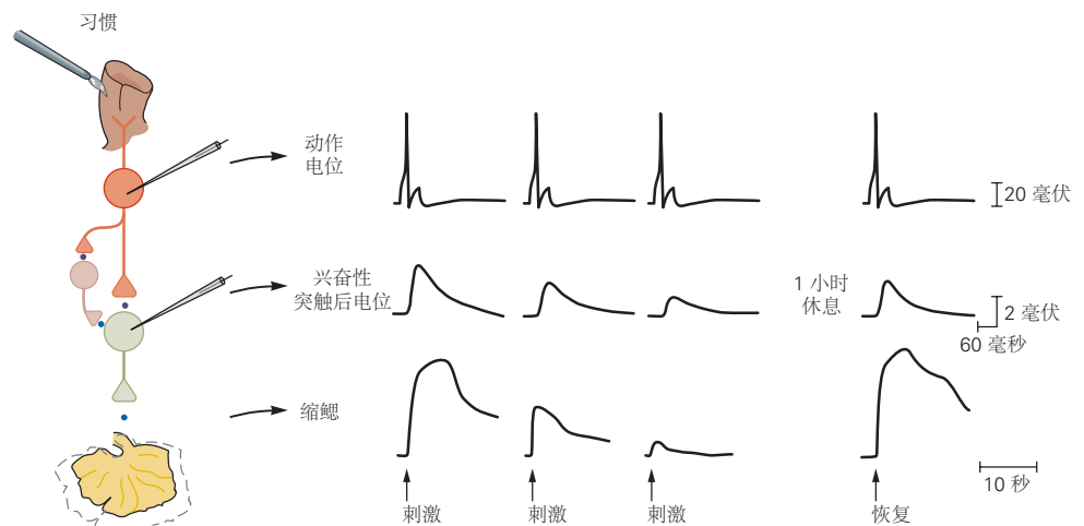
图 53.1.1: 海蜗牛海兔的缩鳃反射的短期习惯。A. 海兔的背视图展示了呼吸器官（鳃）和外套膜，它以虹吸管结束，虹吸管是一种用于排出海水和废物的肉质喷口。触摸虹吸管会引起缩鳃反射。反复刺激会导致习惯。B. 缩鳃反射回路和习惯化部位的简化图。腹部神经节中大约 24 个机械受体神经元支配虹吸管皮肤。这些感觉细胞在支配鳃的 6 个运动神经元以及调节运动神经元放电的中间神经元上形成兴奋性突触（为简单起见，此处仅说明了每种类型的神经元中的一个）。触摸虹吸管会导致缩鳃（虚线轮廓显示原始鳃大小；实线轮廓显示最大退缩）。C. 反复刺激虹吸管感觉神经元（顶部痕迹）导致感觉神经元和运动神经元之间的突触传递逐渐抑制。尽管突触前动作电位没有变化，但运动神经元兴奋性突触后电位的大小逐渐减小。在一个单独的实验中，虹吸管的反复刺激导致鳃退缩（习惯化）的减少。重复刺激一小时后，兴奋性突触后电位和退缩都已恢复。习惯化涉及整个反射回路中许多突触位点的递质释放减少 [496] 。
