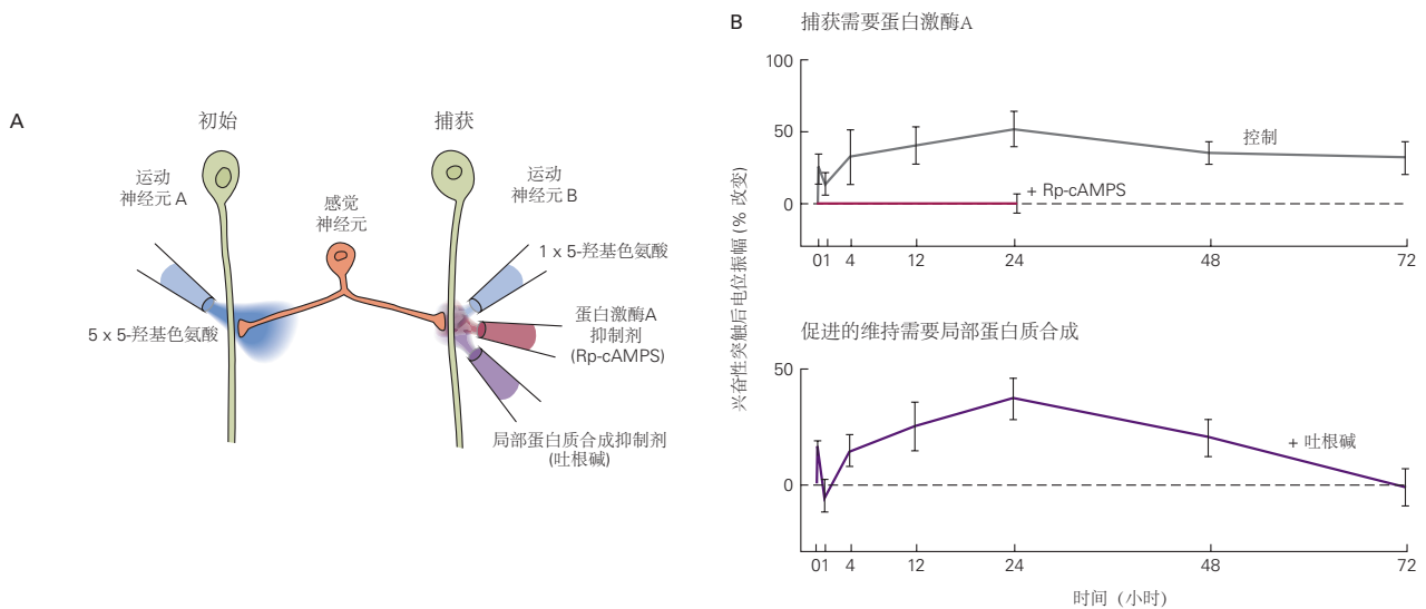
图 53.2.6: 长期促进需要环磷酸腺苷依赖性磷酸化和局部蛋白质合成 [503] 。A. 5 个 5-羟基色氨酸脉冲应用于运动神经元 A 的突触，单脉冲应用于细胞 B 的突触。蛋白质抑制剂（蛋白激酶 A；Rp-cAMPS）或局部蛋白质合成（吐根碱）应用于细胞 B 上的突触。B. Rp-cAMPS 在神经元 B 的突触处完全阻断长期易化作用的捕获。吐根碱对捕获、促进或新突触连接的增长在 5-羟基色氨酸应用后 24 小时测量，但到 72 小时，它完全阻止突触增强。新突触连接的产物被缩回，如果局部蛋白质合成不维持捕获，则长期促进会在 1 天后衰减。
