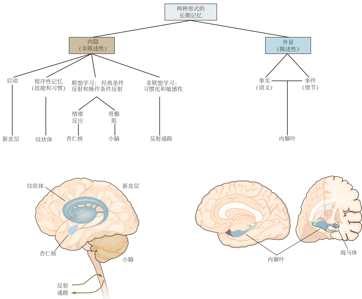
图 53.0.1: 2 种形式的长期记忆涉及不同的大脑系统。内隐记忆涉及新皮层、纹状体、杏仁核、小脑，在最简单的情况下，还涉及反射通路本身。外显记忆需要内侧颞叶和海马体，以及新皮层的某些区域（未显示）。
