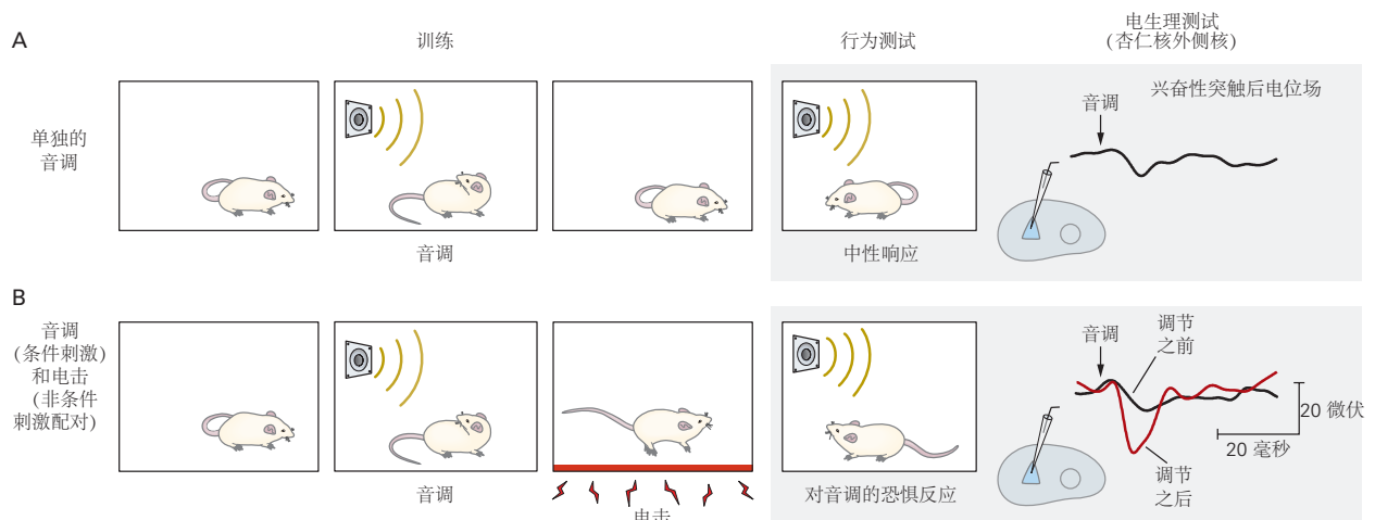
图 53.4.2: 威胁学习会产生相关的行为和电生理变化。A. 动物通常会忽略中性音调。音调在细胞外场电极记录的杏仁核中产生小的突触响应。当兴奋性突触电流进入大量杏仁核神经元的树突时，杏仁核中的记录电极与大脑外部的第二电极之间的小电压降会产生兴奋性突触后电位场。B. 当音调在足部电击前立即出现时，动物学会将音调与电击联系起来。结果，单是音调就会引起先前引起的震惊：它会导致老鼠僵滞，这是一种本能的防御响应。威胁条件反射后，杏仁核外侧核对音调的电生理响应大于条件反射前的响应 [506] 。
