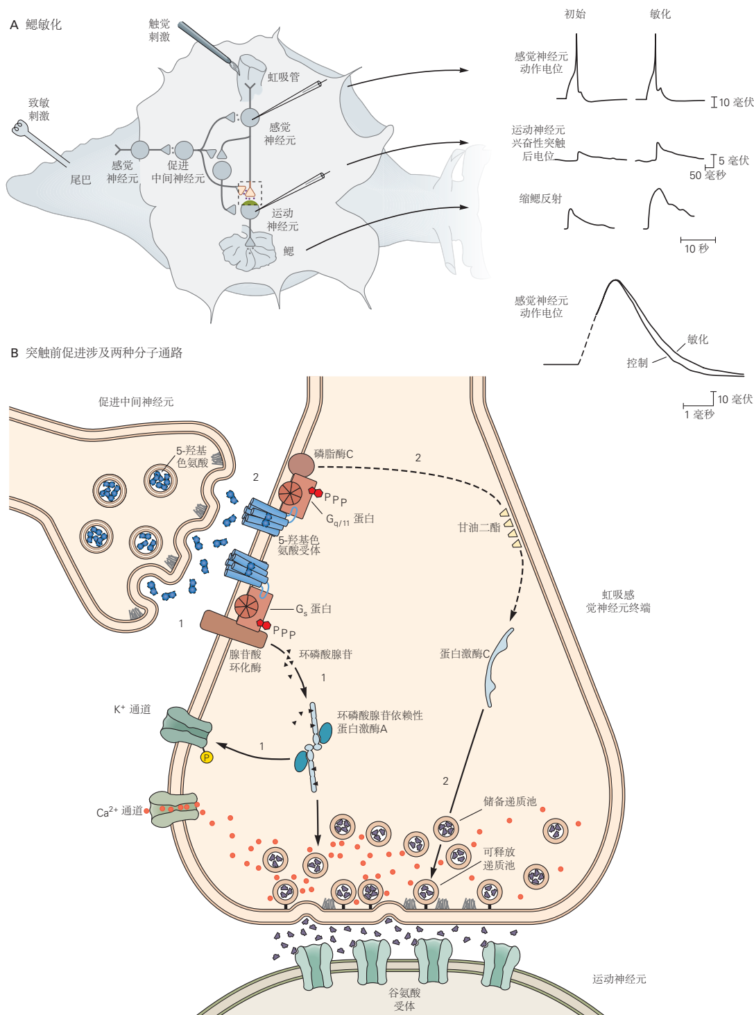
图 53.1.3: 海兔缩鳃反射的短期敏化。A. 对身体的另一部分 (例如尾巴) 施加伤害性刺激会产生缩鳃反射。对尾部的电击会激活尾部感觉神经元, 从而激发促进 (调节) 中间神经元, 从而在支配虹吸管的机械受体感觉神经元的细胞体和末端形成突触。通过这些轴-轴突触, 调节中间神经元增强递质从虹吸感觉神经元释放到它们的突触后鳃运动神经元 (突触前易化), 从而增强鳃退缩。突触前易化部分是由感觉神经元动作电位 (底部轨迹) 的延长引起的 [496,498] 。B. 感觉神经元中的突触前易化作用被认为是通过 2 种生化通路发生。该图在 A 部分的虚线框中显示了突触复合体的详细信息。通路 1: 促进中间神经元释放 5-羟基色氨酸, 它与感觉神经元末梢的促代谢受体结合。该作用与 G 蛋白 ( G_s ) 结合, 进而增加腺苷酸环化酶的活性。腺苷酸环化酶将三磷酸腺苷转化为环磷酸腺苷, 后者与蛋白激酶 A 的调节亚基结合, 从而激活其催化亚基。催化亚基磷酸化某些 K^+ 通道, 从而关闭通道并减少向外的 K^+ 电流。这会延长动作电位, 从而增加 Ca^{2+} 通过电压门控 Ca^{2+} 通道的流入, 从而增加递质释放。通路 2: 5-羟基色氨酸与第二类促代谢受体结合, 后者激活 G 蛋白的 G_{q/11} 类, 从而增强磷脂酶 C 的活性。磷脂酶 C 活性导致甘油二酯的产生, 从而激活蛋白激酶 C。蛋白激酶 C 磷酸化突触前蛋白, 导致含有谷氨酸的囊泡从储备池动员到活性区的可释放池, 从而提高递质释放的效率。
