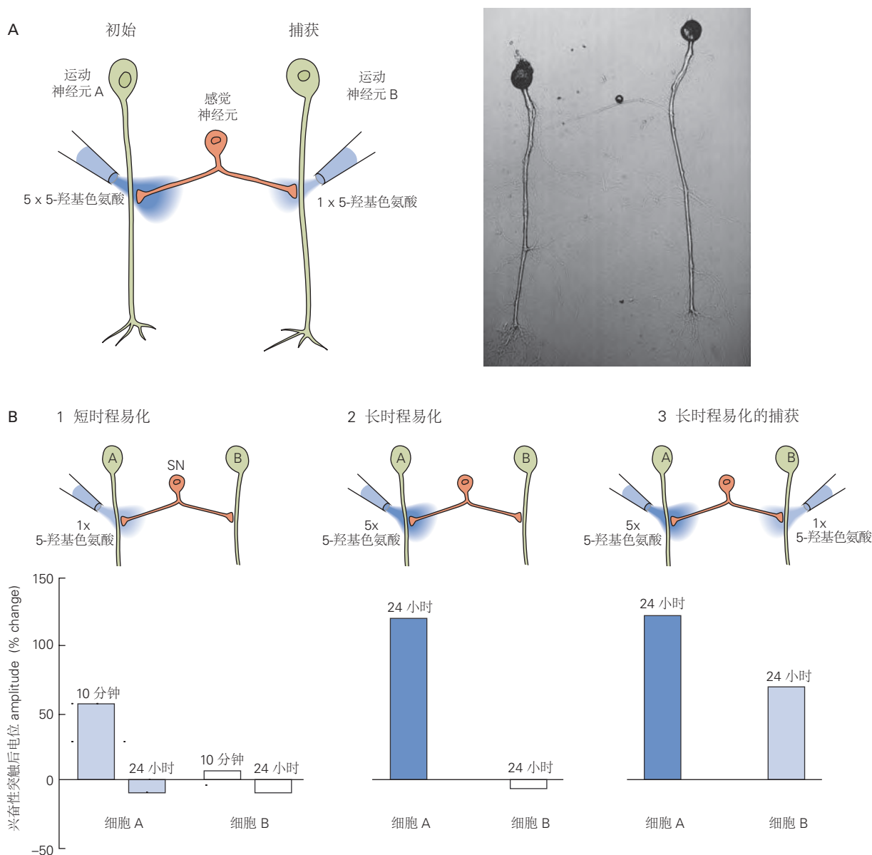
图 53.2.5: 突触传递的长期促进是突触特异性的 [502] 。A. 该实验使用单个突触前感觉神经元与 2 个突触后运动神经元 A 和 B 接触。左侧的吸管用于施加 5 个 5-羟基色氨酸脉冲与运动神经元 A 的感觉神经元突触，在该突触处启动长期促进作用。右侧的吸管用于将 5-羟基色氨酸的一个脉冲施加到具有运动神经元 B 的感觉神经元突触，使该突触能够利用（捕获）细胞体内产生的新蛋白质在与运动神经元 A 的突触处以响应 5-羟基色氨酸的 5 个脉冲。右图显示了培养细胞的实际外观。B. 1. 对运动神经元 A 的突触施加 1 个 5-羟基色氨酸脉冲，仅对神经元中的兴奋性突触后电位产生短期（10 分钟）促进作用。24 小时后，兴奋性突触后电位已恢复到正常大小。细胞 B 中的兴奋性突触后电位大小没有显著变化。2. 对细胞 A 的突触施加 5 次 5-羟基色氨酸脉冲会对该细胞中的兴奋性突触后电位产生长期（24 小时）促进作用，但不会影响细胞 B 中的兴奋性突触后电位大小。3. 当对细胞 A 的突触施加 5 次 5-羟基色氨酸脉冲和对细胞 B 施加 1 次 5-羟基色氨酸脉冲时，细胞 B 现在显示长期促进和增加 24 小时后以兴奋性突触后电位大小。
