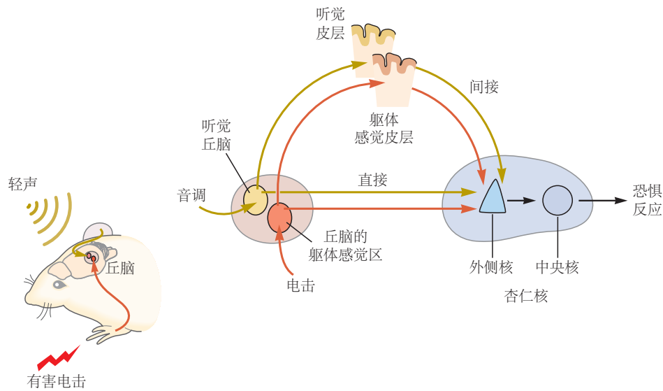
图 53.4.1: 威胁学习涉及从丘脑到杏仁核的并行通路。条件刺激的信号（此处是中性音调）通过两条通路从听觉丘脑传递到杏仁核外侧核：通过直接通路和通过听觉皮层的间接通路。类似地，无条件刺激的信号（这里是电击）通过并行的伤害感受通路从丘脑的体感部分传递到外侧核：一个是直接通路，一个是通过体感皮层的间接通路。外侧核依次投射到中央核，即杏仁核的输出核，它激活神经回路，增加心率，产生其他自主神经变化，并引发构成防御状态的防御行为 [505] 。
