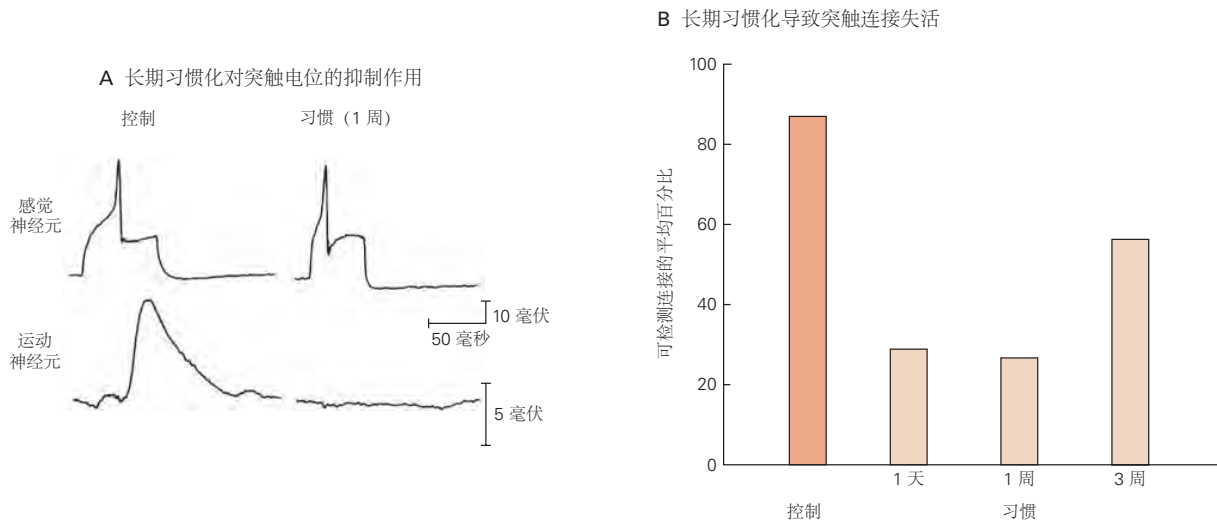
图 53.1.2: 海兔缩鳃反射的长期习惯 [497] 。A. 未受训动物（对照）和长期习惯动物的感觉神经元动作电位和运动神经元突触后电位的比较。在训练后 1 周的习惯动物中，运动神经元中没有响应感觉神经元动作电位的突触电位。B. 经过长期的习惯训练，即使在 3 周时，与运动神经元建立生理可检测连接的感觉神经元的平均百分比也会降低。
