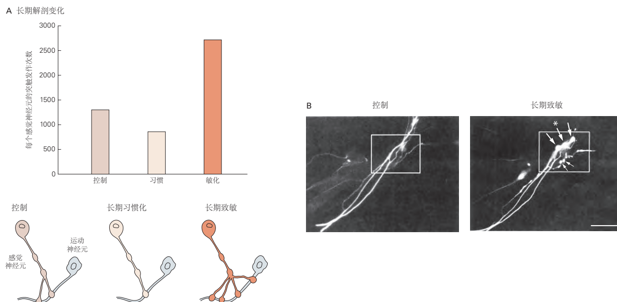
图 53.2.4: 长期习惯化和敏化涉及感觉神经元突触前末梢的结构变化。A. 长期习惯导致突触丢失，长期致敏导致突触数量增加。当在训练后 1 天（此处显示）或 1 周进行测量时，相对于对照水平，致敏动物的突触前末梢数量较多，而习惯动物较少。图表下方的图说明了突触接触数量的变化。感觉神经元突起上的肿胀或静脉曲张称为突触神经节；它们包含递质释放所需的所有专用结构 [500] 。B. 接触培养物中的运动神经元的轴突在 5 次短暂暴露于 5-羟色胺之前（左）和之后 1 天（右）的荧光图像。由此产生的静脉曲张增加模拟了与长期致敏相关的突触变化。在应用 5-羟色胺之前，在轮廓区域（左）中看不到突触前静脉曲张。在 5-羟色胺之后，几个新的扣结是显而易见的（箭头），其中一些包含完全发育的活性区（星号）或具有小的未成熟活性区。比例尺 = 50 微米 [501] 。
