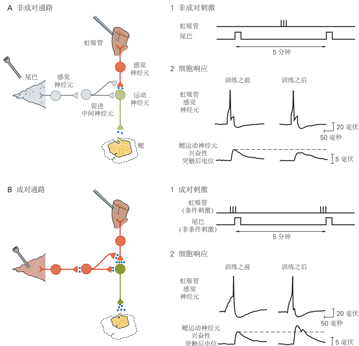
图 53.1.4: 海兔缩鳃反射的经典调节 [499] 。A. 虹吸管受到轻敲刺激，尾巴受到电击，但 2 种刺激没有及时配对。尾部电击会刺激促进中间神经元，在感觉神经元的突触前末梢形成突触，这些中间神经元会在支配外套膜和虹吸管的神经元的突触前末梢形成突触。这就是致敏机制。1. 训练过程中不成对刺激的模式。2. 在这些条件下，运动神经元测试兴奋性突触后电位的大小仅受尾部电击的微弱影响。通常，如本例所示，尽管存在尾部电击，但兴奋性突触后电位实际上会略有下降，因为虹吸管的重复不成对刺激会因习惯而导致突触抑制。B. 尾部电击与虹吸管的刺激及时配对。1. 在电击尾巴（非条件刺激）之前立即触摸虹吸管（条件刺激）。结果，虹吸管感觉神经元准备好对来自无条件通路中的易化中间神经元的输入更敏感。这是经典条件反射的机制；它选择性地放大条件通路的响应。2. 在训练前和训练后 1 小时由虹吸感觉神经元产生的已识别运动神经元中测试兴奋性突触后电位的记录。在使用配对感觉输入进行训练后，虹吸运动神经元中的兴奋性突触后电位比训练前的兴奋性突触后电位或未配对的尾部电击后的兴奋性突触后电位大得多（如 A2 部分所示）。这种突触放大会产生更有力的鳃收缩。
