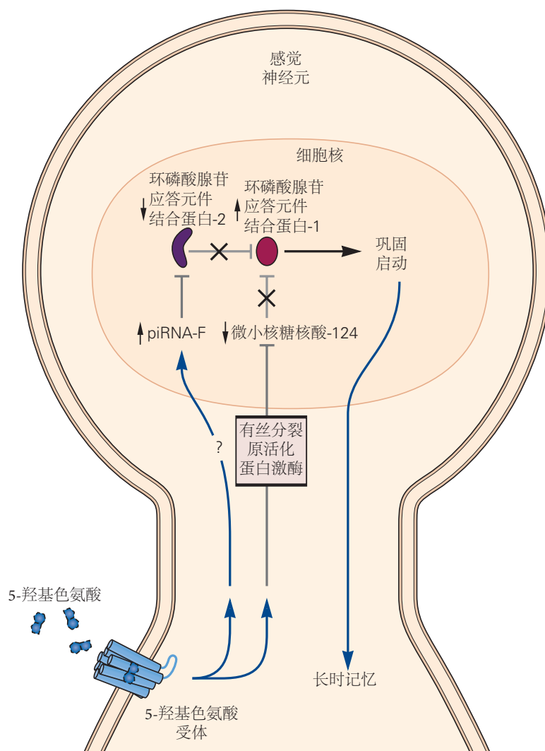
图 53.2.3: 小的非编码核糖核酸分子有助于记忆巩固开关。通过 2 种不同类别的小非编码核糖核酸分子的作用，巩固了感觉运动神经元突触的长期促进作用。微小核糖核酸-124 通常通过与其信使核糖核酸结合并抑制其翻译来抑制环磷酸腺苷应答元件结合蛋白-1 转录因子的水平。5-羟基色氨酸通过需要有丝分裂原活化蛋白激酶的机制下调微小核糖核酸-124 水平。这提高了环磷酸腺苷应答元件结合蛋白-1 的水平，促进了记忆巩固所必需的基因产物的环磷酸腺苷应答元件结合蛋白-1 依赖性转录的激活。在互补通路中，5-羟基色氨酸增强并延迟了几种与 Piwi 蛋白相作用的核糖核酸的合成，包括与 Piwi 蛋白相作用的核糖核酸-F。与 Piwi 蛋白相作用的核糖核酸-F/ Piwi 复合物导致环磷酸腺苷应答元件结合蛋白-2 基因的甲基化增强，导致环磷酸腺苷应答元件结合蛋白-2 的长期转录抑制和环磷酸腺苷应答元件结合蛋白-2 蛋白水平降低。由于环磷酸腺苷应答元件结合蛋白-2 通常会抑制环磷酸腺苷应答元件结合蛋白-1 的作用，因此响应 5-羟基色氨酸的与 Piwi 蛋白相作用的核糖核酸-F 水平增加会增强和延长环磷酸腺苷应答元件结合蛋白-1 活性，从而导致更有效的记忆巩固。
