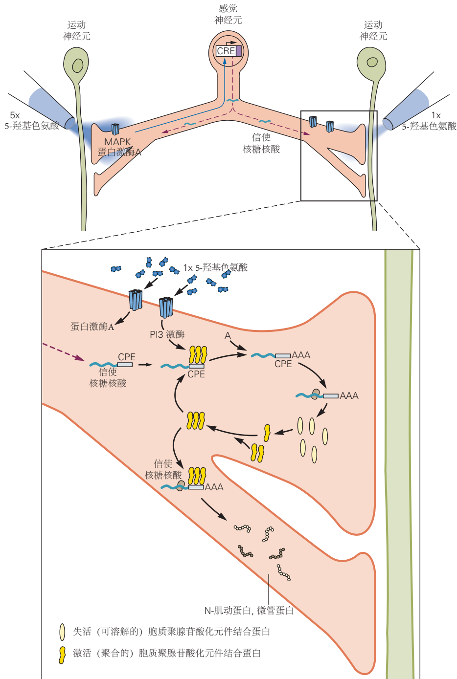
图 53.2.7: 海兔轴突末梢蛋白质合成的自我延续开关可维持长期突触促进。5 个 5-羟基色氨酸脉冲会产生 1 个信号，该信号会返回细胞核以激活信使核糖核酸的合成。然后通过快速轴突运输将细胞体中新转录的信使核糖核酸和新合成的蛋白质发送到所有终端。然而，只有那些被至少 1 个 5-羟基色氨酸脉冲标记的终端才能使用这些蛋白质来生长长期促进所需的新突触。终端的标记涉及 2 种物质：(1) 蛋白激酶 A，它是运输到终端的蛋白质启动的即时突触生长所必需的，以及 (2) 磷酸肌醇 3-激酶，它启动维持突触生长和超过 24 小时的长期促进所需的信使核糖核酸的局部翻译。末端的一些信使核糖核酸编码胞质聚腺苷酸化元件结合蛋白，这是一种局部蛋白质合成的调节剂。在基础状态下，胞质聚腺苷酸化元件结合蛋白被认为以一种基本无活性的构象存在，作为一种不能与信使核糖核酸结合的可溶性单体。通过 5-羟基色氨酸和磷酸肌醇 3-激酶激活的一些尚未明确的机制，胞质聚腺苷酸化元件结合蛋白的一些拷贝转化为形成聚集体的活性构象。聚集体的功能类似于朊病毒，因为它们能够募集单体加入聚集体，从而激活单体。胞质聚腺苷酸化元件结合蛋白聚集体结合信使核糖核酸的胞质聚腺苷酸化元件位点。这种结合会募集多 A 聚合酶机制，并允许将腺嘌呤核苷酸 (A) 的多 A 尾添加到休眠的信使核糖核酸中。多聚腺苷酸化的信使核糖核酸现在可以被核糖体识别，从而允许将这些信使核糖核酸翻译成几种蛋白质。例如，除了胞质聚腺苷酸化元件结合蛋白之外，这还会导致 N-肌动蛋白和微管蛋白的局部合成，从而稳定新生长的突触结构 [504] 。
