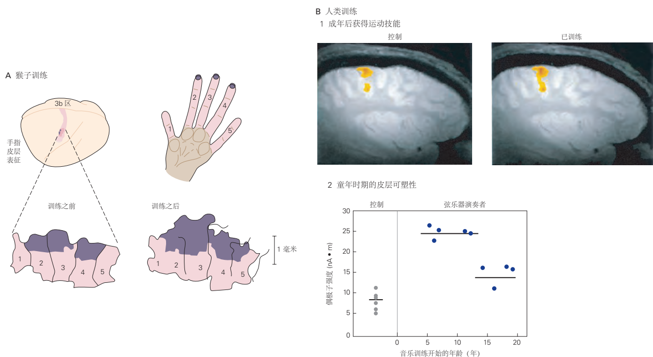
图 53.5.1: 训练扩展了大脑皮层中手指输入的代表。A. 一只猴子每天接受 1 小时的训练，以执行一项需要重复使用指尖 2、3 和偶尔使用 4 的任务。训练后，体感皮层 3b 区中代表受刺激手指指尖的部分（深色）明显大于正常值（训练前 3 个月测量） [510] 。B. 1. 经过 3 周的日常训练（每天 10-20 分钟），受过快速手指运动序列训练的人类受试者将提高准确性和速度。训练后初级运动皮层的功能性核磁共振成像扫描（基于局部血氧水平依赖信号）显示，受过训练的受试者（橙色区域）激活的区域大于未受过训练（对照）的激活区域。对照组受试者未接受任何训练，并使用与对照组受试者相同的手进行未学习的手指运动。受过训练的受试者皮层表征的变化持续了几个月。2. 弦乐演奏者的左手小指皮层代表的大小比非音乐家大。该图绘制了从脑磁图获得的偶极子强度，脑磁图是神经活动的一种测量方法。这种增长在 13 岁之前开始接受音乐训练的音乐家中最为明显 [511] 。
