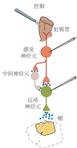
图 53.1.1: 海蜗牛海兔的缩鳃反射的短期习惯。A. 海兔的背视图展示了呼吸器官（鳃）和外套膜，它以虹吸管结束，虹吸管是一种用于排出海水和废物的肉质喷口。触摸虹吸管会引起缩鳃反射。反复刺激会导致习惯。B. 缩鳃反射回路和习惯化部位的简化图。腹部神经节中大约 24 个机械受体神经元支配虹吸管皮肤。这些感觉细胞在支配鳃的 6 个运动神经元以及调节运动神经元放电的中间神经元上形成兴奋性突触（为简单起见，此处仅说明了每种类型的神经元中的一个）。触摸虹吸管会导致缩鳃（虚线轮廓显示原始鳃大小；实线轮廓显示最大退缩）。C. 反复刺激虹吸管感觉神经元（顶部痕迹）导致感觉神经元和运动神经元之间的突触传递逐渐抑制。尽管突触前动作电位没有变化，但运动神经元兴奋性突触后电位的大小逐渐减小。在一个单独的实验中，虹吸管的反复刺激导致鳃退缩（习惯化）的减少。重复刺激一小时后，兴奋性突触后电位和退缩都已恢复。习惯化涉及整个反射回路中许多突触位点的递质释放减少 [496] 。
