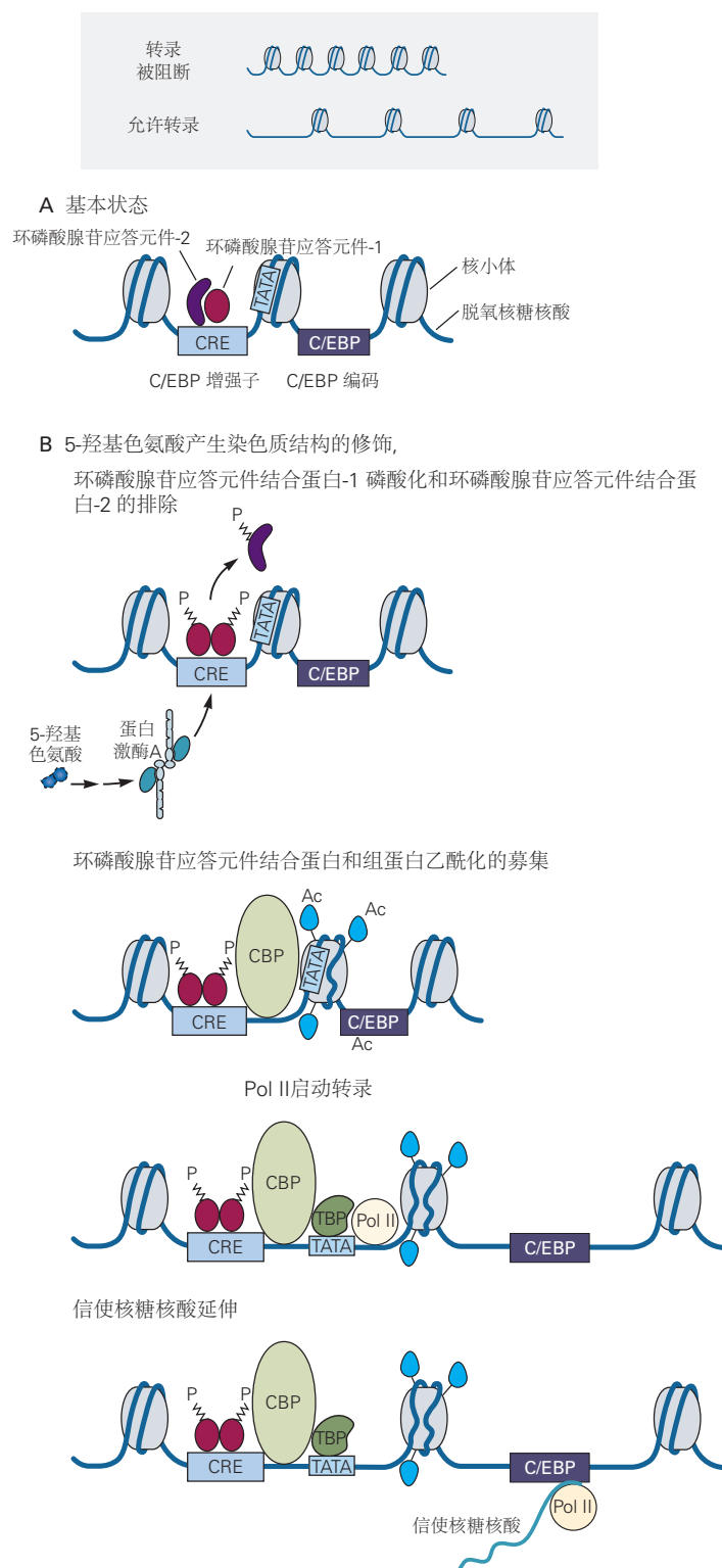
图 53.2.2: 5-羟色氨酸、环磷酸腺苷应答元件结合蛋白-1 和环磷酸腺苷应答元件结合蛋白对组蛋白乙酰化的调节。 A. 在基础条件下，激活剂 环磷酸腺苷应答元件结合蛋白-1（此处与 环磷酸腺苷应答元件结合蛋白-2 复合）占据其靶基因启动子区域内环磷酸腺苷应答元件的结合位点。在此处显示的示例中，环磷酸腺苷应答元件结合蛋白-1 与 C/EBP 启动子内的环磷酸腺苷应答元件结合。在基础状态下，环磷酸腺苷应答元件结合蛋白-1 结合无法激活转录，因为 TATA 盒是转录起始期间负责募集核糖核酸聚合酶 II（Pol II）的核心启动子区域，无法进入，因为脱氧核糖核酸与组蛋白紧密结合核小体。B. 5-羟色氨酸激活蛋白激酶 A，使 环磷酸腺苷应答元件结合蛋白-1 磷酸化并通过 有丝分裂原活化蛋白激酶间接增强 环磷酸腺苷应答元件结合蛋白-2 磷酸化，导致 环磷酸腺苷应答元件结合蛋白-2 从启动子上解离。这允许 环磷酸腺苷应答元件结合蛋白-1 在启动子处与 环磷酸腺苷应答元件结合蛋白结合蛋白形成复合物。活化的环磷酸腺苷应答元件结合蛋白乙酰化组蛋白的特定赖氨酸残基，导致它们与脱氧核糖核酸的结合不那么紧密。随着染色质结构的其他变化，乙酰化有助于核小体的重新定位，该核小体先前阻止了 Pol II 复合物进入 TATA 盒。这种重新定位允许募集 Pol II 以启动 C/EBP 基因的转录。
