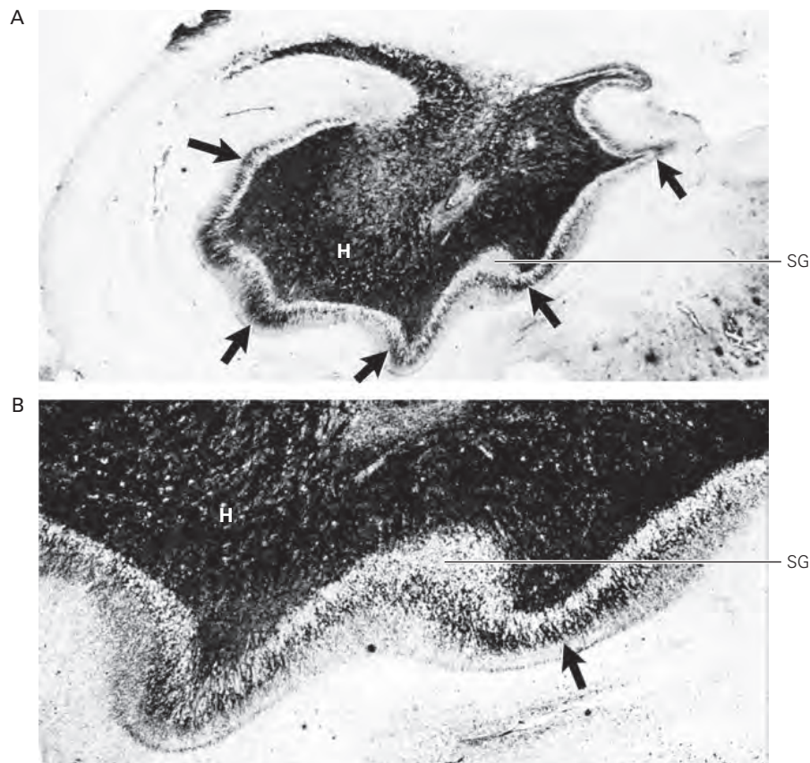
图 58.7.2: 人类颞叶的苔藓纤维突触重组（发芽）可能导致过度兴奋 [556] 。A. 癫痫患者在颞叶切除术控制癫痫时切除的海马横截面的 Timm 染色。齿状颗粒细胞（苔藓纤维）的轴突中出现黑色染色，这是由于这些轴突中存在锌。苔藓纤维通常通过齿状门（H）到达阿蒙角 3 锥体细胞上的突触。在这里显示的癫痫组织中，染色纤维出现在齿状回（SG，箭头）的颗粒上层，该层现在不仅包含颗粒细胞树突，还包含新发芽的苔藓纤维。这些苔藓纤维的异常芽在齿状颗粒细胞上形成新的反复兴奋性突触。B. 颗粒上层的高倍镜更详细地显示了 Timm 染色的苔藓纤维。
