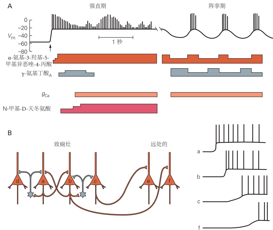
图 58.3.3: 局灶性发作开始于后超极化和周围抑制的丧失 [552] 。A. 随着发作的开始（箭头），发作灶中的神经元去极化，就像阵发性去极化转变的第一阶段一样。然而，与发作间期不同的是，去极化持续数秒或数分钟。 \gamma -氨基丁酸介导的抑制作用失败，而 \alpha -氨基-3-羟基-5-甲基-4-异恶唑丙酸- 和 N-甲基-D-天冬氨酸型谷氨酸受体的兴奋性在功能上增强。这种活动对应于继发性全身性强直阵挛发作的强直期。随着 \gamma -氨基丁酸介导的抑制逐渐恢复，癫痫病灶中的神经元进入与阵挛期相对应的振荡期。B. 随着周围抑制的瓦解，癫痫病灶中的神经元同步兴奋，并向远处的神经元发送一系列动作电位，从而从病灶传播异常活动。如图 58.3.2B 所示，将细胞 a 到 c 中的这种活动模式与发作间期的活动模式进行比较。
