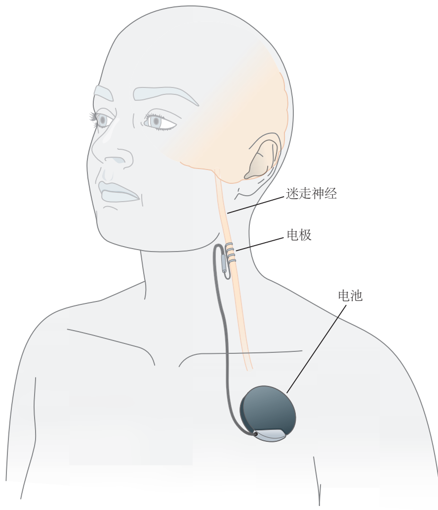
图 58.3.4: 迷走神经刺激。电极在左迷走神经上的放置示意图，由皮下植入胸壁的电 池供电。刺激可以按规则的间隔（例如，每 30 秒）进行编程，也可以根据需要在胸部放置磁铁来激活 [553] 。
