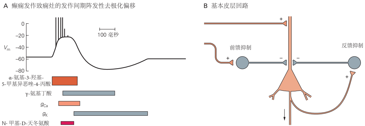
图 58.3.1: 癫痫病灶中神经元阵发性去极化转变的电导。A. 阵发性去极化偏移在很大程度上取决于 \alpha -氨基-3-羟基-5-甲基-4-异恶唑丙酸和 N-甲基-D-天冬氨酸-型谷氨酸受体-通道, 其有效性通过电压门控 \text{Ca}^{2+} 通道 ( g_{\text{Ca}} ) 的打开而增强。去极化后, 细胞通过激活 \gamma -氨基丁酸受体 (离子型 \gamma -氨基丁酸 A 和代谢型 \gamma -氨基丁酸 B ) 以及电压门控和钙激活 \text{K}^{+} 通道 ( g_{\text{K}} ) 而超极化 [552] 。B. 反复出现的轴突分支激活抑制性神经元并引起锥体神经元的反馈抑制。外在兴奋性输入也可以激活前馈抑制。阵发性去极化偏移代表癫痫病灶中的过度兴奋, 而抑制回路构成环绕抑制的基础, 对于将发作间期活动限制在癫痫病灶中很重要。
