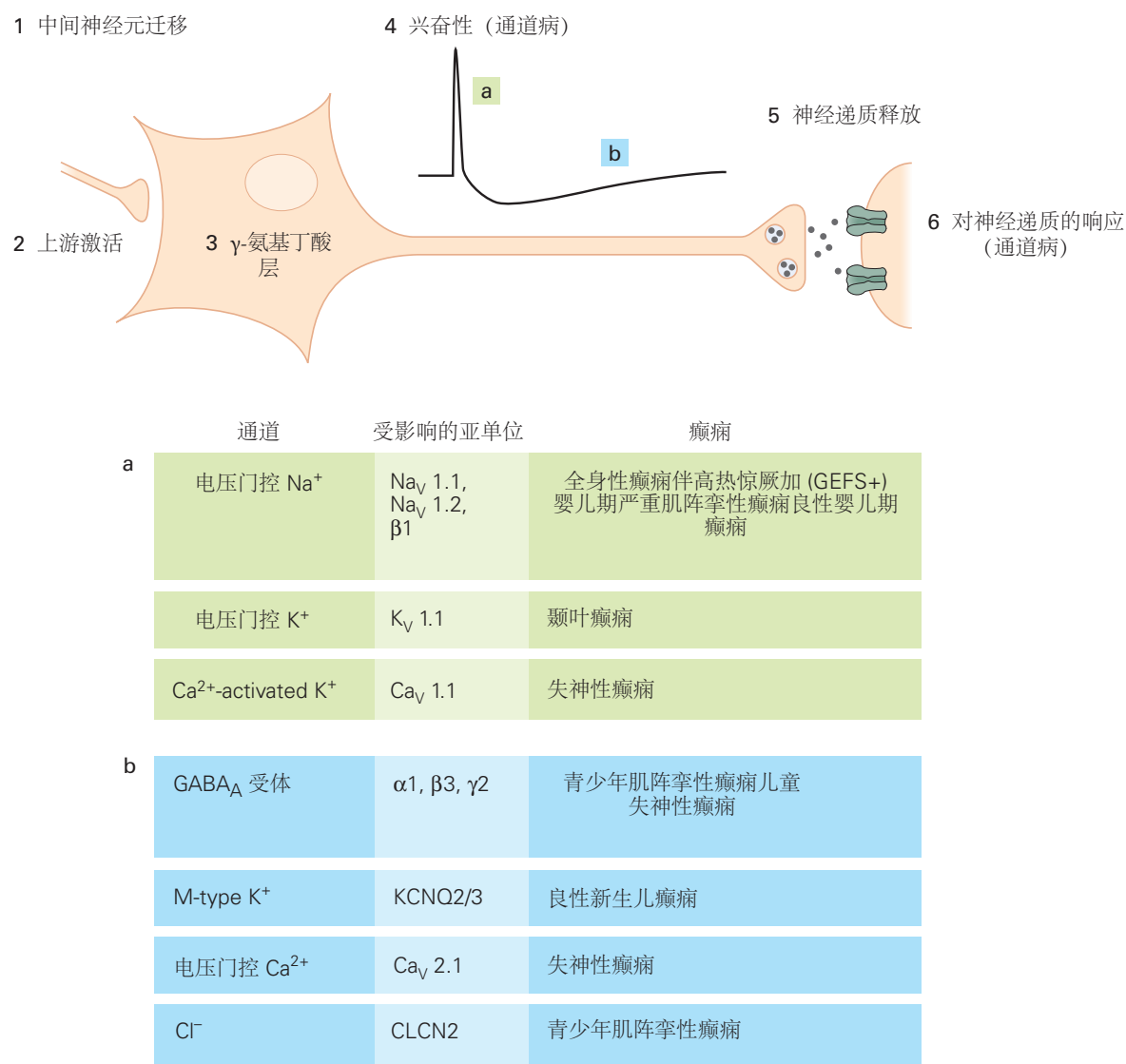
图 58.7.1: 离子通道病是单基因人类癫痫的主要原因，但不是唯一原因。迄今为止发现的人类癫痫基因可以影响突触传递的多个阶段，包括中间神经元的迁移 (1)、中间神经元的上游激活 (2)、中间神经内的 \gamma -氨基丁酸水平 (3)、兴奋性和抑制性神经元的兴奋性 (4)、神经递质的释放 (5) 以及对神经递质的突触后响应 (6)。插图显示，这些基因突变对神经元兴奋性的影响可以影响动作电位的形状以及随后的后电位和突触事件。脉冲 (a) 附近显示的突变影响动作电位的复极。(b) 中所示的其他突变影响后超极化、突触传导或棘间间隔。
