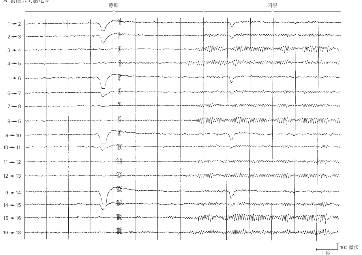
图 58.2.1: 觉醒人类受试者的正常脑电图。A. 头皮表面的一组标准电极放置位置 (或蒙太奇)。每个位置的电响应反映了 2 个电极之间的活动。B. 在记录开始时, 脑电图显示头皮表面存在低电压活动 (20 微伏)。垂直线以 1 秒为间隔放置。在最初的 8 秒内, 受试者睁着眼睛静静地休息, 然后要求受试者闭上眼睛。闭眼时, 枕骨区域 (位点 3、4、8、12、15 和 16) 会出现更大幅度的活动 (8–10 赫兹)。这是放松、觉醒状态的正常 \alpha 节律特征。眨眼时 3.5 秒和闭眼时 9 秒时会出现缓慢的大振幅伪影。
