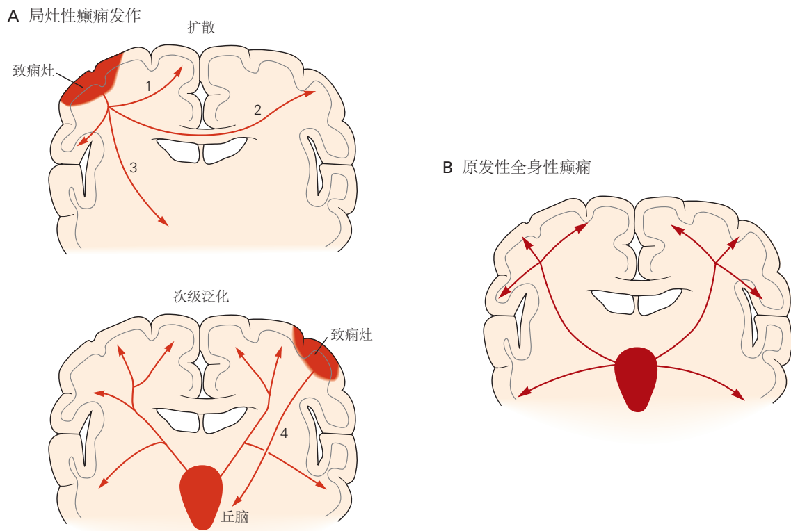
图 58.3.6: 局灶性和全身性发作通过多种通路传播 [555] 。A. 局灶性癫痫发作可以通过大脑半球内纤维 (1) 从病灶局部扩散，并更远处扩散至等位对侧皮层 (2) 和皮层下中心 (3)。局灶性癫痫发作的继发性泛化通过投射到丘脑扩散到皮层下中心 (4)。广泛的丘脑皮层互连随后有助于 2 个半球的快速激活。B. 在全身性癫痫发作中，例如典型的失神性癫痫，丘脑和皮层之间的相互联系是癫痫发作传播的主要通路。
